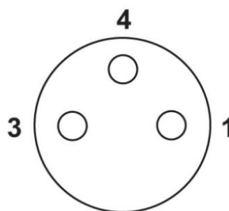
Schaltplan
