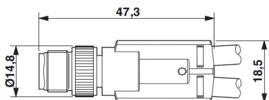
Maßzeichnung, M12Y Steckverbinder
