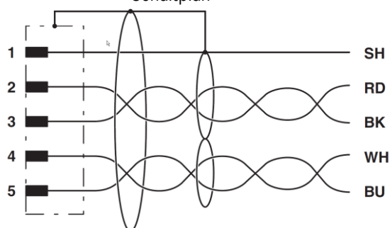
Schaltplan
