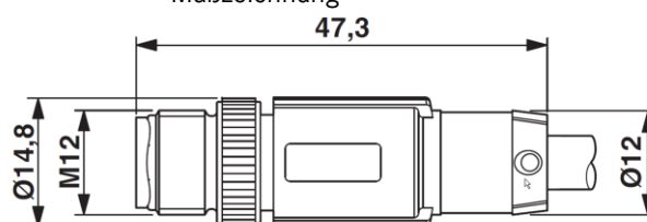
Maßzeichnung
