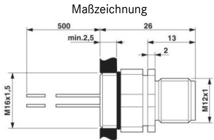
M12-Einbaubuchse, positionierbar
