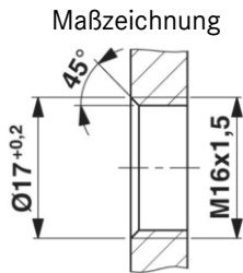
Gehäuseausschnitt für M16-Befestigungsgewinde, Montagewand mit Gewinde
