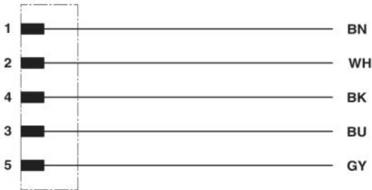
Kontaktbelegung des M12-Steckers und der M12-Buchs
