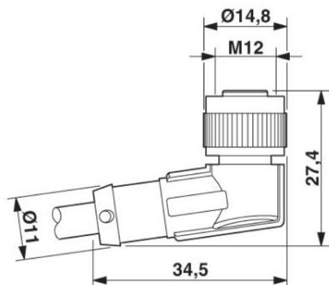
Maßzeichnung, M12 Steckverbinder
