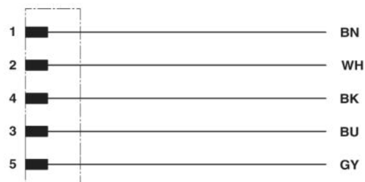
Schaltplan
