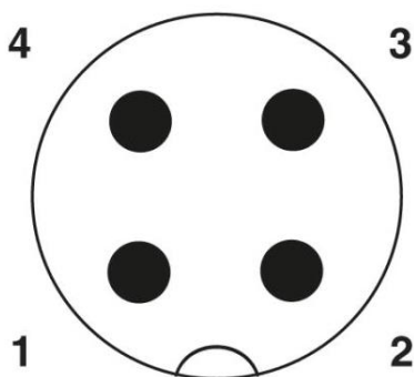
Schaltplan
