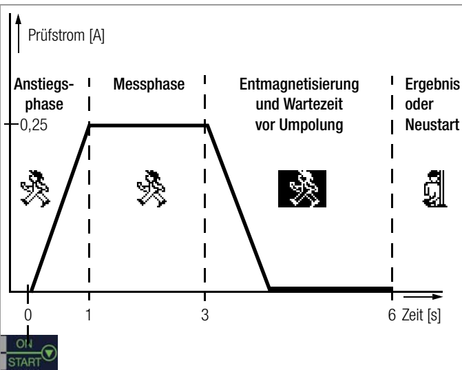
Darstellung der Mess- und Wartephases bei der Schutzleiterwiderstandsmessung an PRCDs mit dem PROFITEST MXTRA
