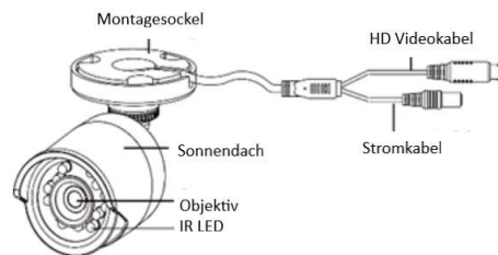
Abbildung 1-1 Kamerakomponenten
