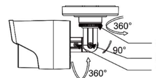
Abbildung 2-3 3-Achsenausrichtung
