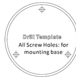
Abbildung 2-1 Bohrschablone
