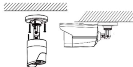
Abbildung 2-2 Kamera befestigen
