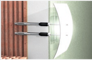
Befestigung von Außenleuchten in Mauerwerk mit dem fisher Thermax
