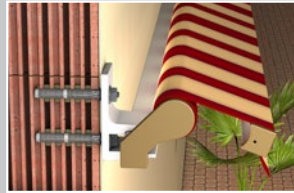
Markisenbefestigung in Mauerwerk mit dem fisher Injektionsmörtel FIS V und der Injektions Ankerhülse FIS H
