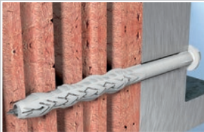
Anwendung in Hochlochziegel mit dem fisher Langschaftdübel SXRL
