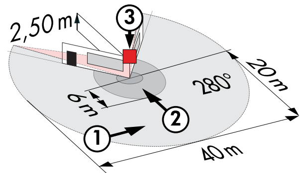
Reichweitendiagramm
