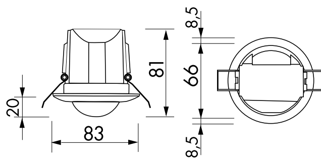
Bemaßung 92184
