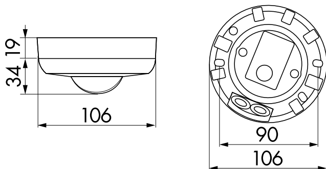
Bemaßung 92219
