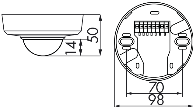
Bemaßung 92550
