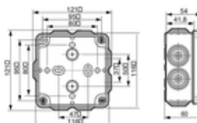
■ Plexo vierkante doos 105 x 105 mm
