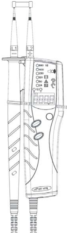
Abb. 6: Durchgangstest
