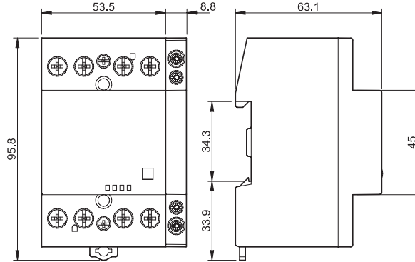
Typ 022.63/022.65 (6 A-Hilfsschalter für 22.44 und 22.64) Schraubklemmen
