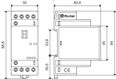
Typ 22.44/22.64 Schraubklemmen
