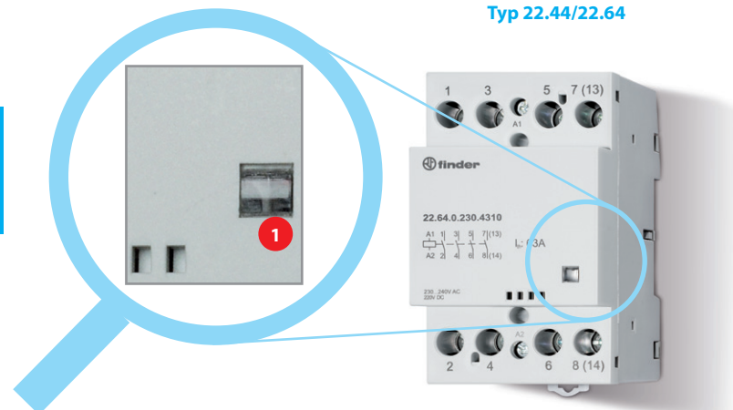
Typ 22.44/22.64
