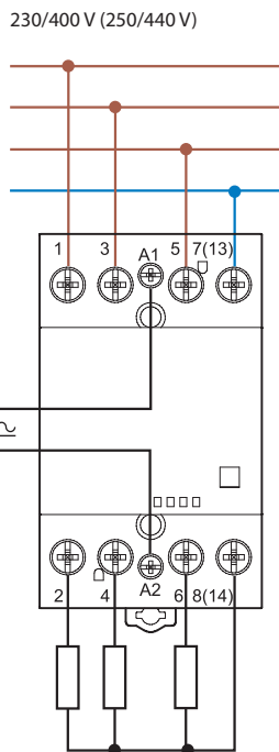
Typ 22.44/22.64
