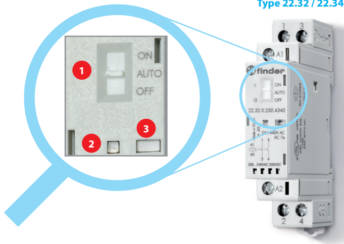
Typ 22.32 / 22.34
