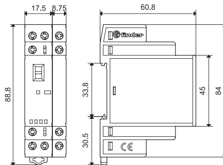
Typ 22.34 + 022.33/022.35 Schraubklemmen
