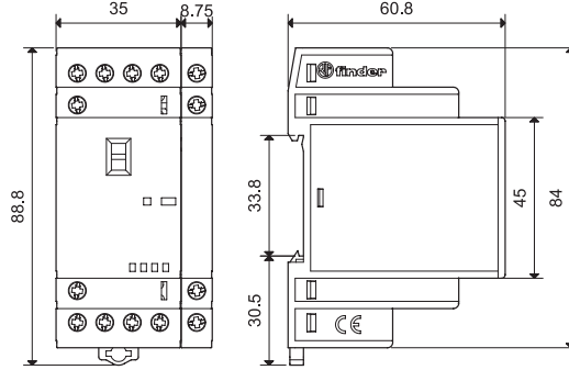
Typ 22.44/22.64 + 022.63/022.65 Schraubklemmen
