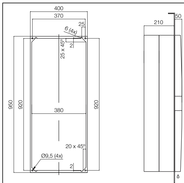
Abb. 108: 3304.xxx, 3305.xxx Kompletteinbau
