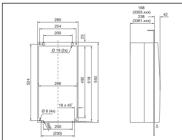
Abb. 107: 3303.xxx, 3361.xxx Kompletteinbau
