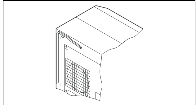
Abb. 7: Dichtungsband ankleben
