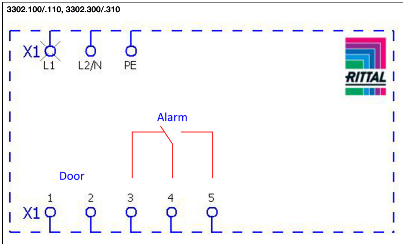
Abb. 23: Elektro-Schaltplan Nr. 1
