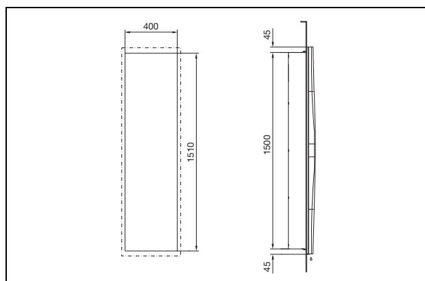
Abb. 110: 3366.xxx Kompletteinbau
