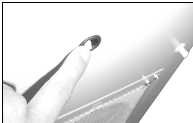
Abb. 62: Displaykabel zurückschieben und durch Kabeldurchführung drücken (2)
