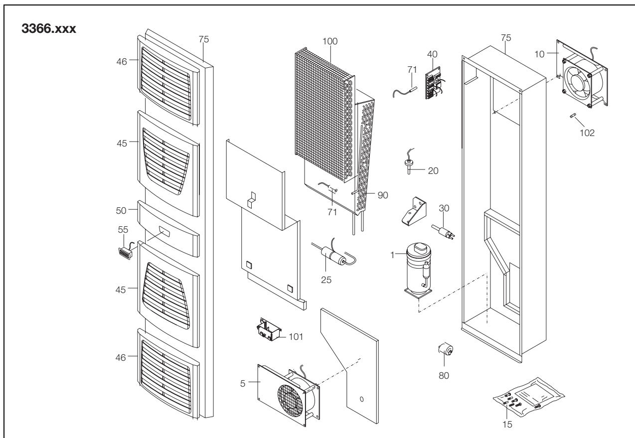
Abb. 90: Ersatzteile 3366.xxx
