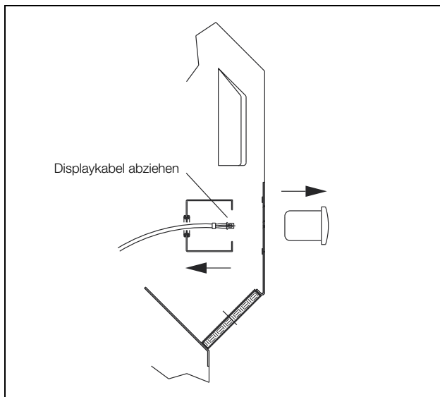
Abb. 81: Demontage Haube (3)
