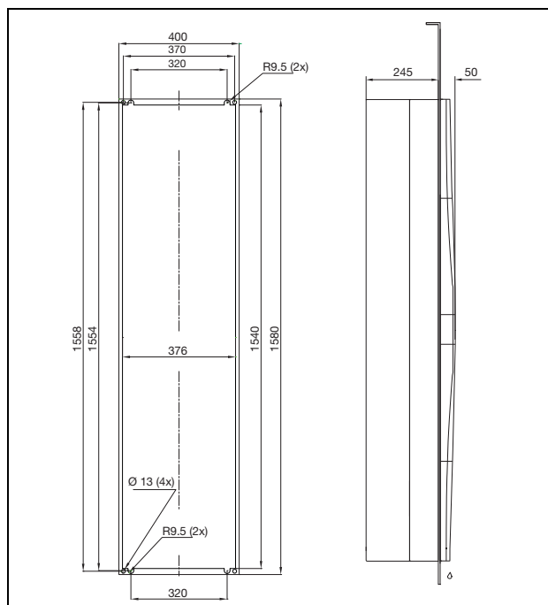
Abb. 109: 3328.xxx, 3329.xxx Kompletteinbau
