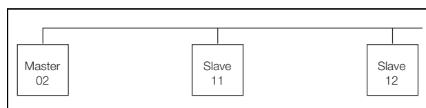
Abb. 33: Master-Slave-Vernetzung (Beispiel)
