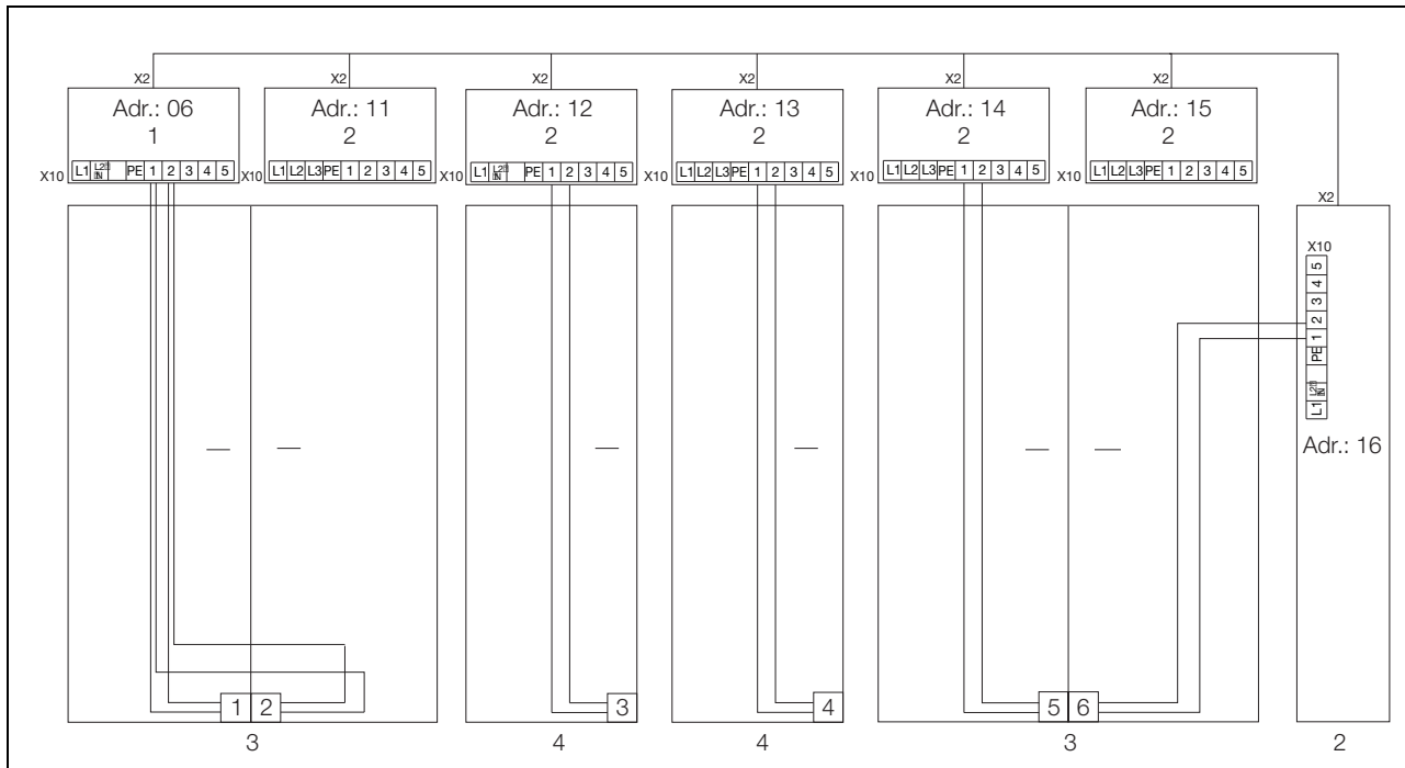
Abb. 22: Anschlussbeispiel: Türendshalter und Master-Slave-Betrieb
