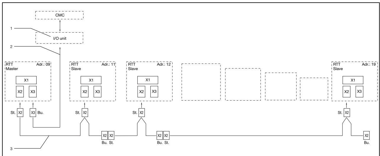
Abb. 21: Anschlussbeispiel: Master-Slave-Betrieb
