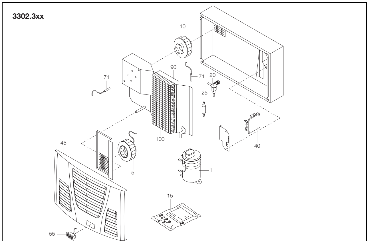
Abb. 85: Ersatzteile 3302.3xx
