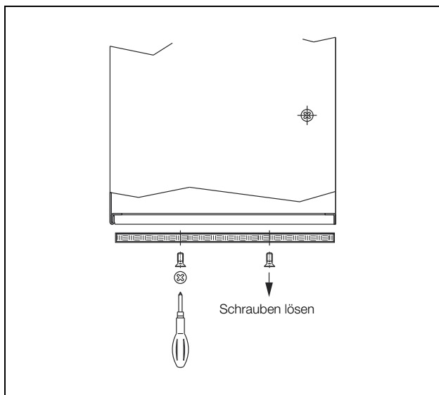
Abb. 82: Filterwechsel
