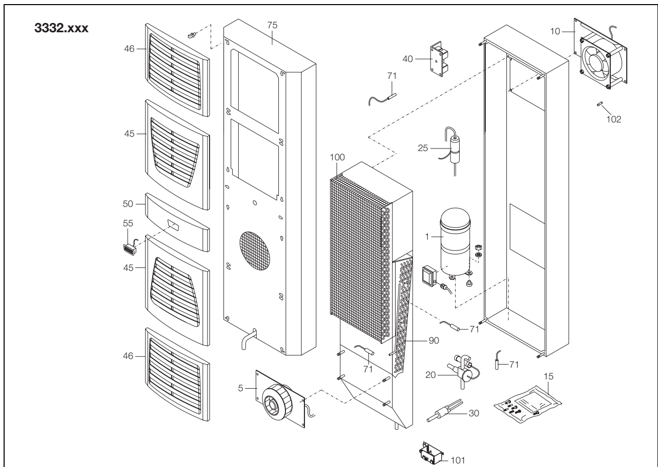
Abb. 89: Ersatzteile 3332.xxx
