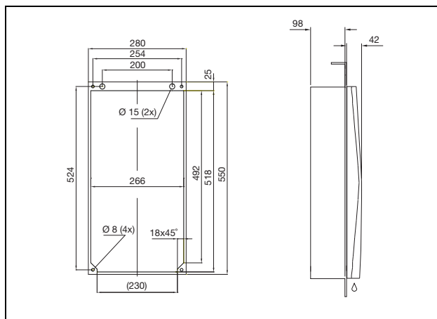
Abb. 105: 3302.xxx Kompletteinbau (außer 3302.3xx)
