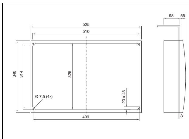
Abb. 106: 3302.3xx Kompletteinbau
