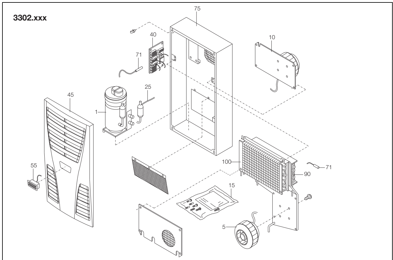
Abb. 84: Ersatzteile 3302.xxx
