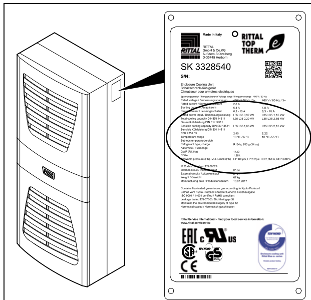
Abb. 83: Typenschild (Technische Daten)
