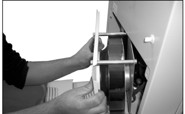
Abb. 42: Lüfter ausbauen
