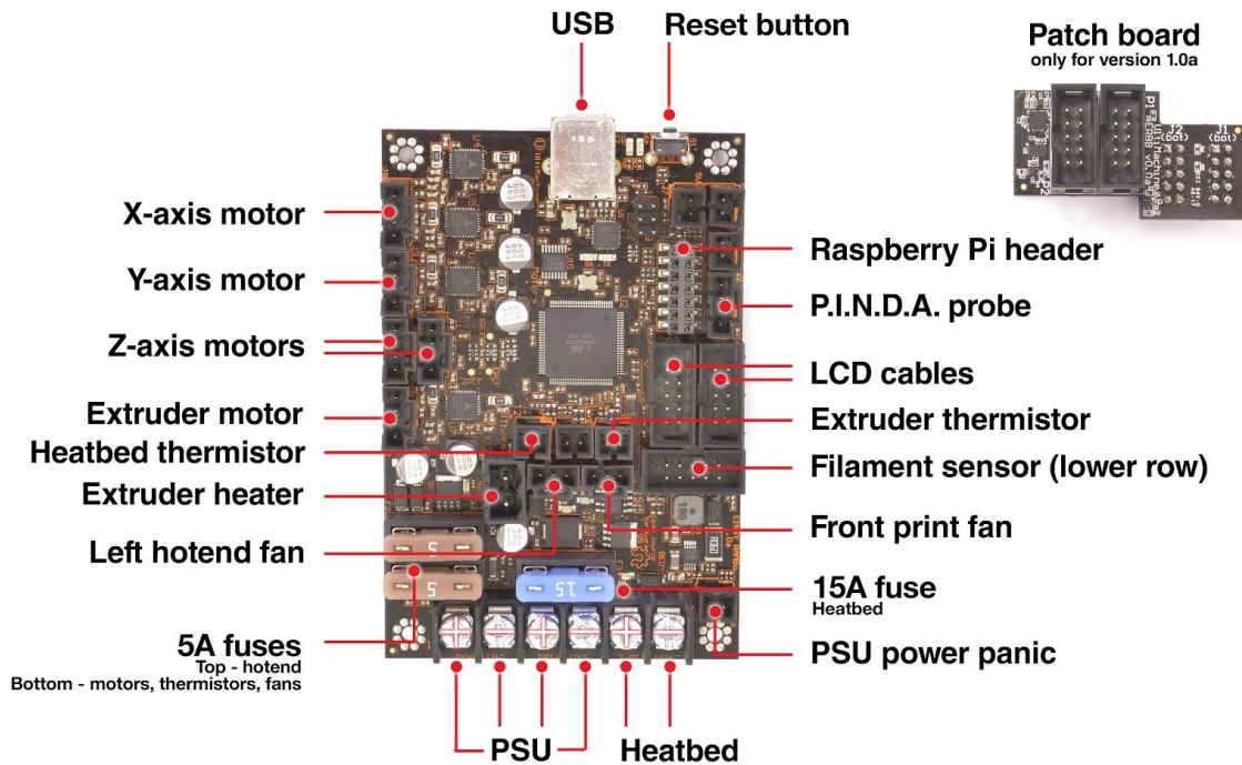
Bild 47 - Korrekte Verdrahtung der Steckverbinder
