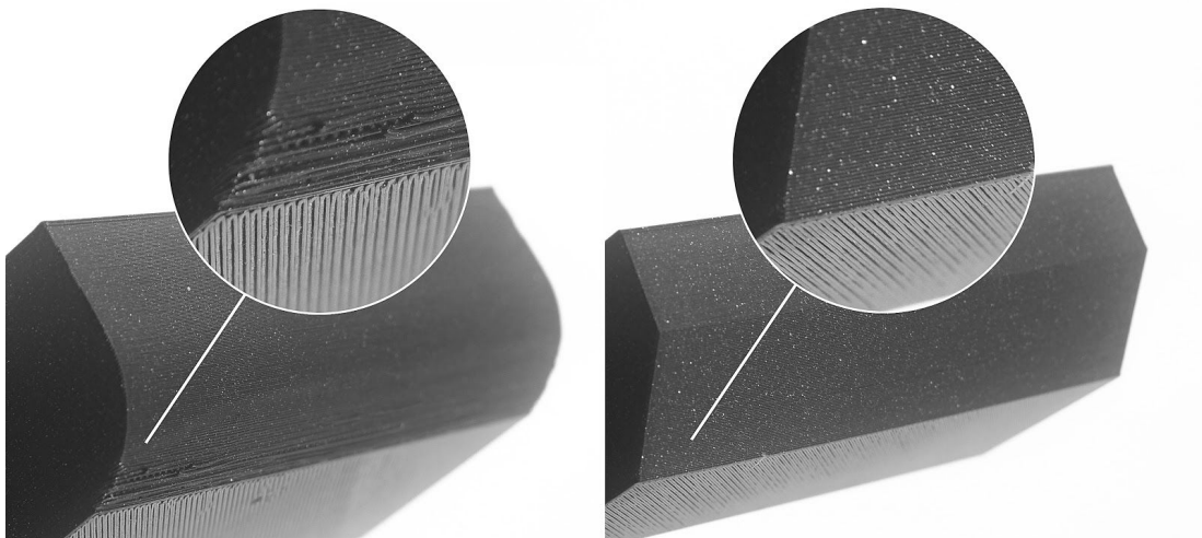
Bild 29 - Verrundung (links) vs. Fase (rechts)
