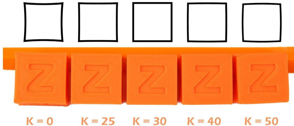
Bild 25 - Wie wirkt sich der K-Wert auf den Druck aus?
