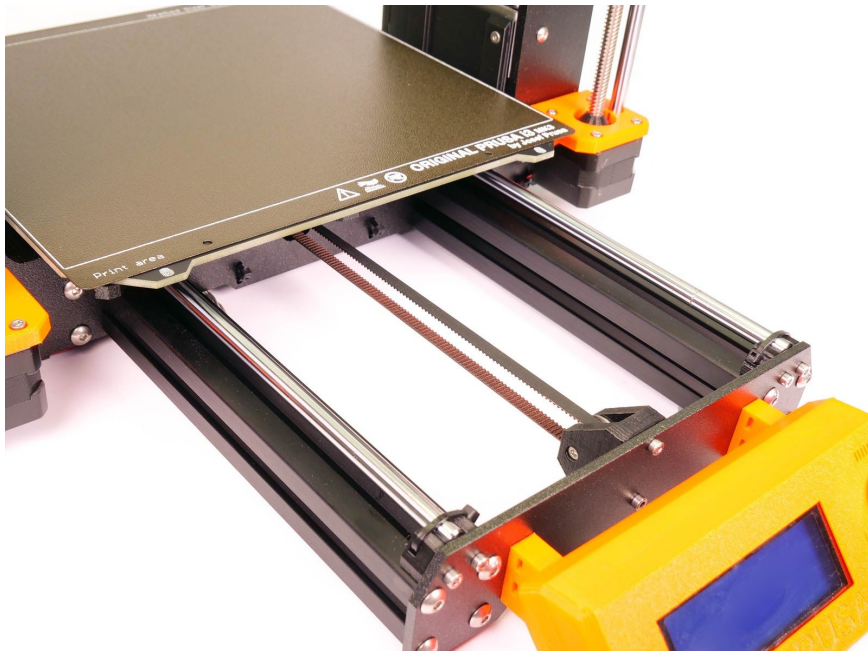
Bild 48 - Ein richtig angezogener Y-Achsenriemen unter dem Heizbett
