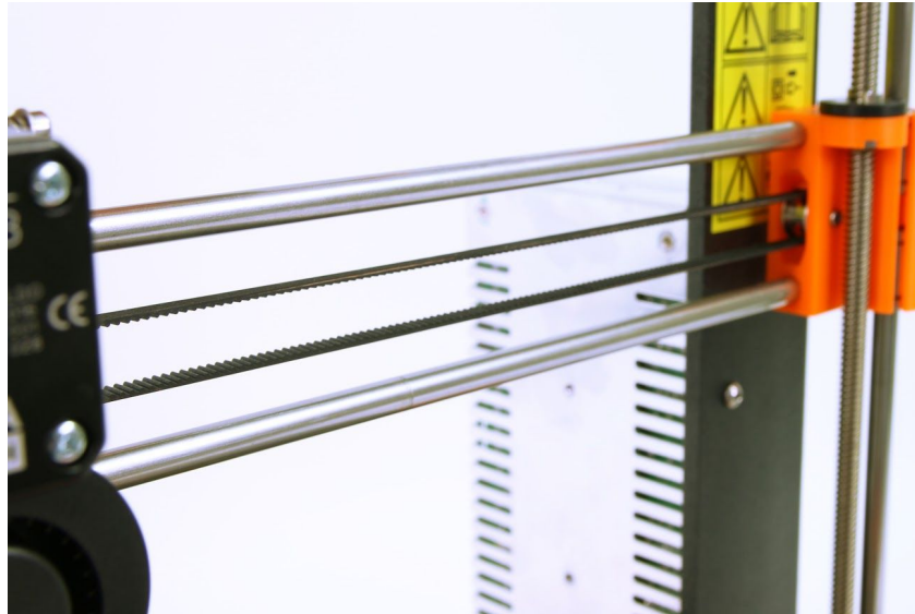
Bild 49 - Ein richtig gespannter X-Achsen-Riemen
