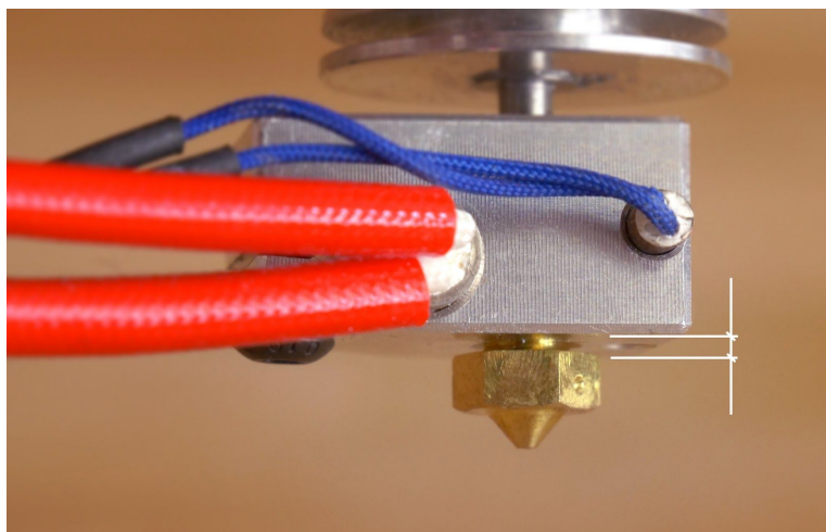
Bild 42 - Ein Spalt zwischen einer vollständig eingeschraubten Düse und dem Heizblock
