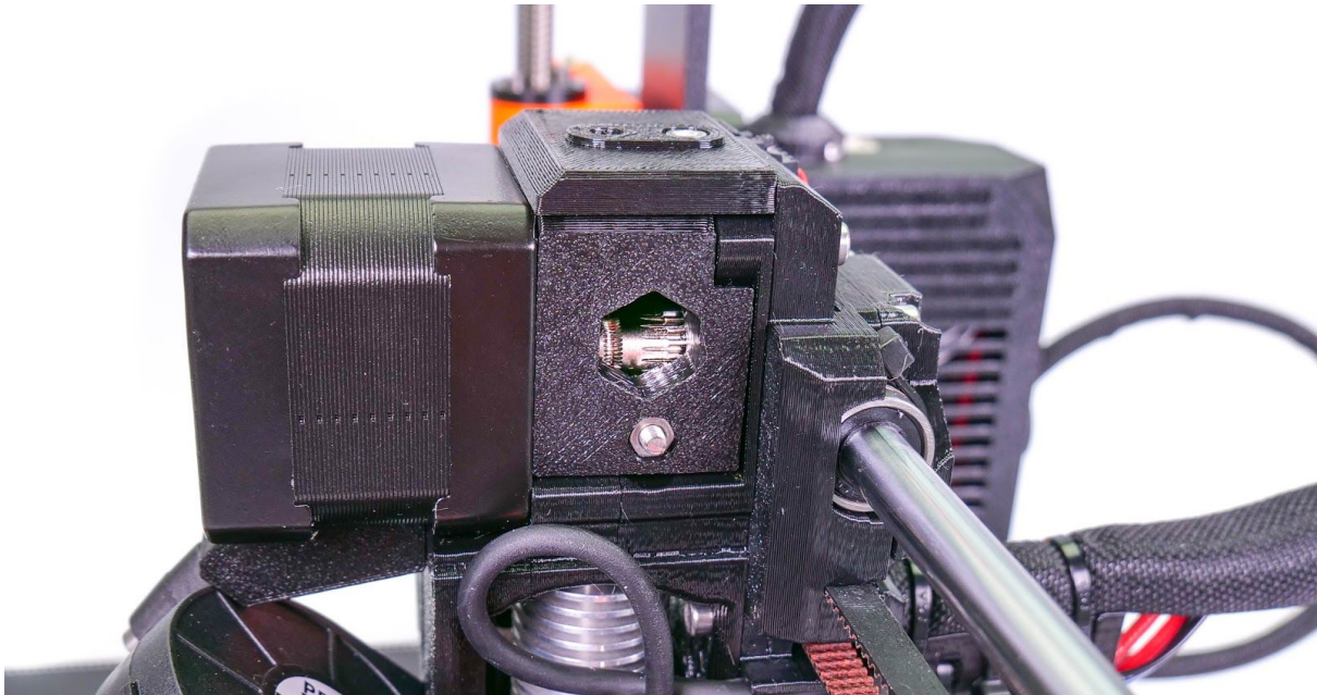
Bild 41 - Reinigen des Extruders - hier sehen Sie die Antriebsritzel durch das Wartungsloch
