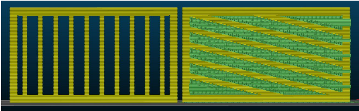
Bild 28 - Modell druckbar ohne Stützen vs. Modell, das viele Stützen benötigt
