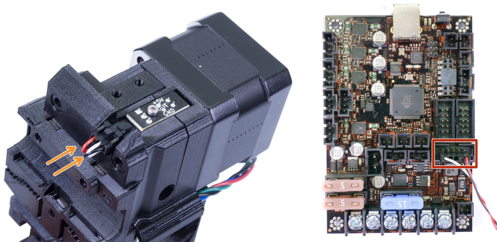
Bild 39 - Korrekt angeschlossener und sitzender Filamentsensor
