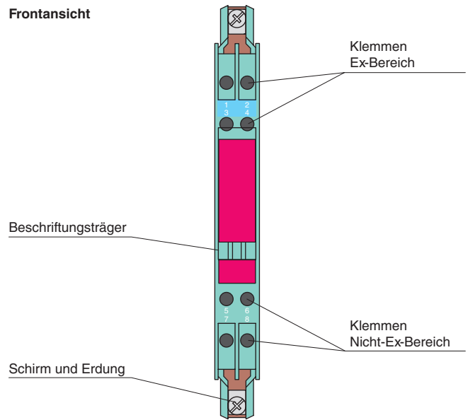
Frontansicht
