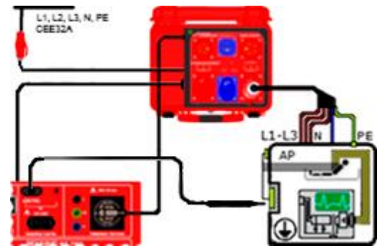
Anschlusschema
