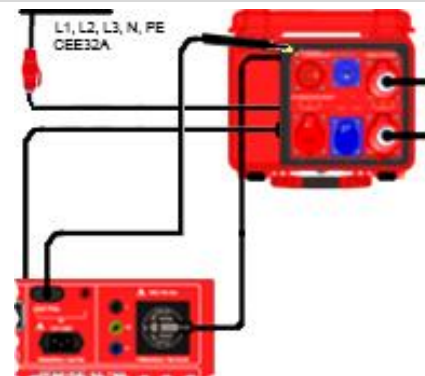
Anschlusschema
