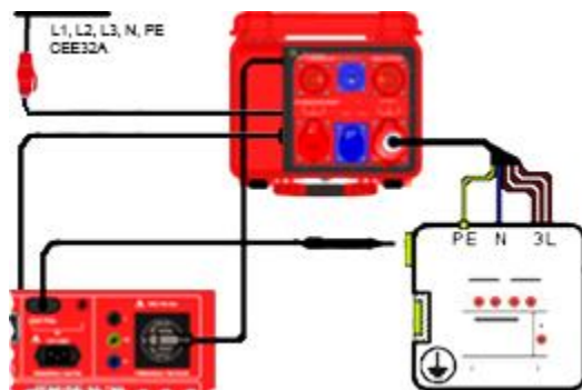
Anschlusschema
