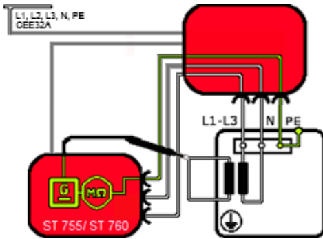
Stromlaufplan
