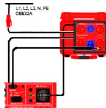
Anschlusschema
