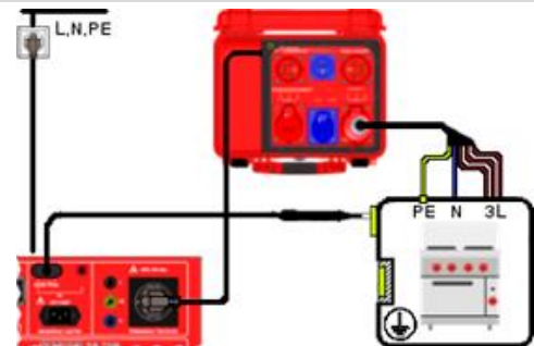
Anschlussschema
