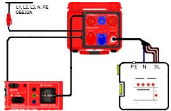
Anschlusschema
