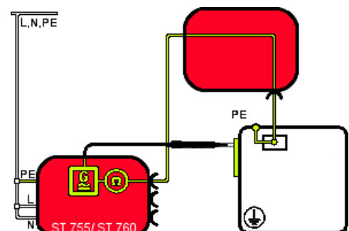
Stromlaufplan
