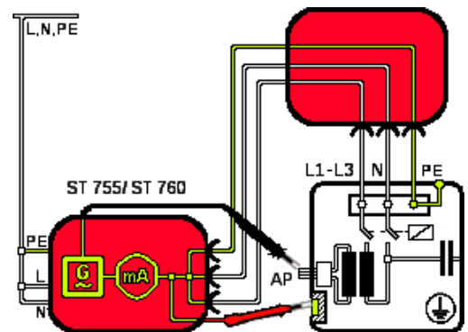
Stromlaufplan
