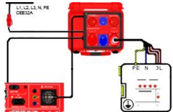
Anschlusschema
