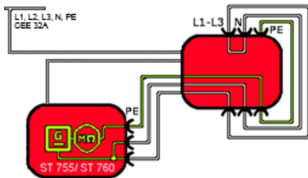
Stromlaufplan
