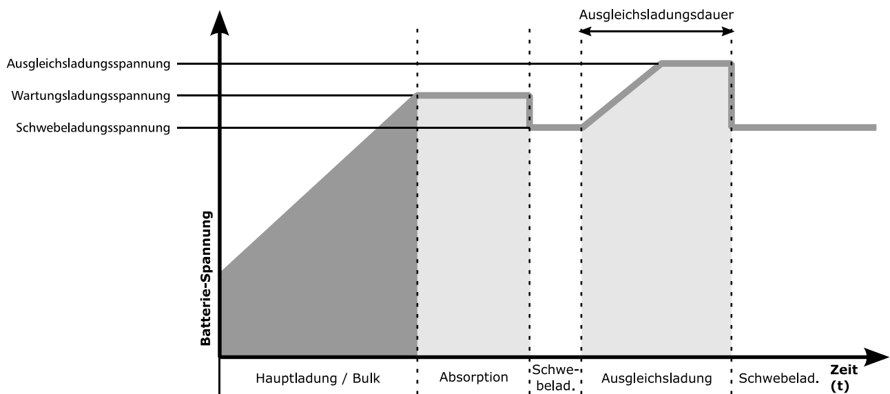
Abbildung 12: ladekurve
