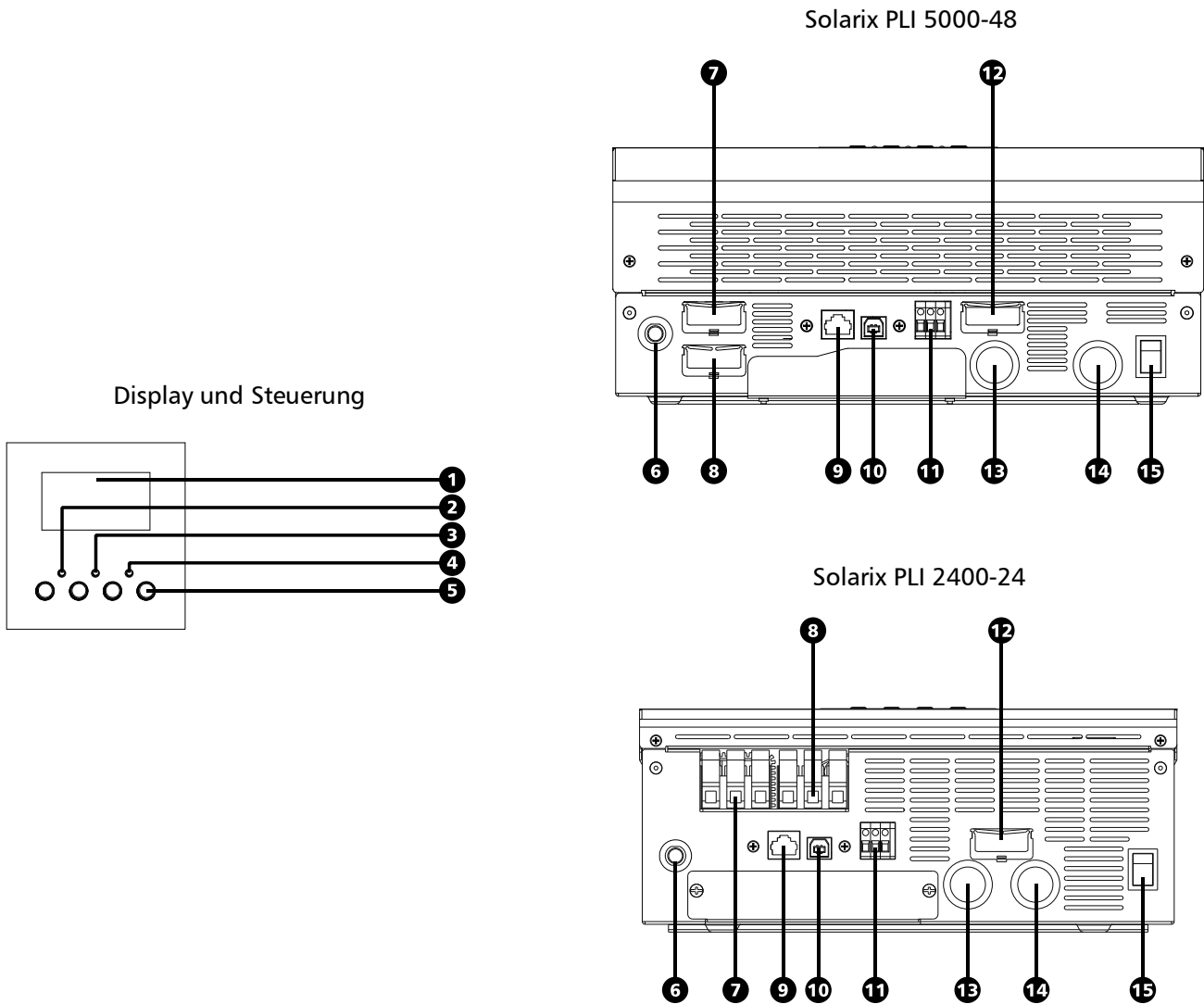
Abbildung 2: Geräteübersicht
