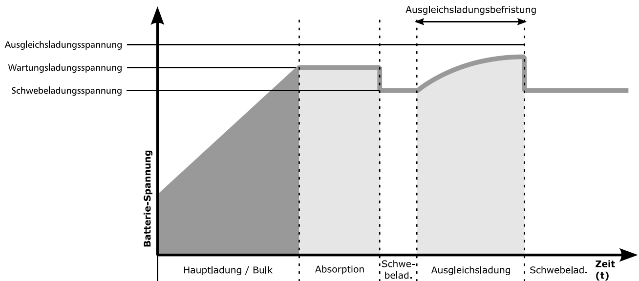
Abbildung 13: Ausgleichladungsbefristung
