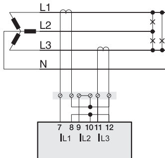
Strommessung über 2 Stromwandler im Dreiphasen-Vierleitersystem
