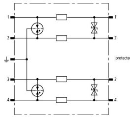
Prinzipialschaltbild BSP M4 BD 24
