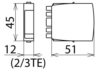
Maßbild BSP M4 BD 24
