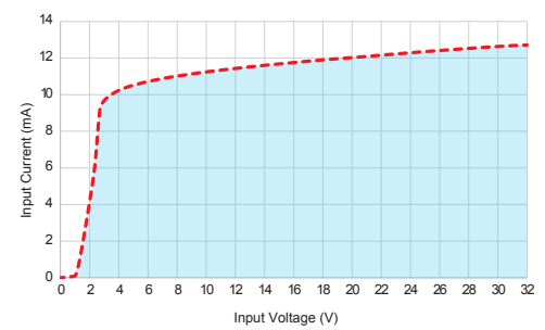
Eingangsstrom vs. Eingangsspannung Standard Geregelte DC-Eingänge
