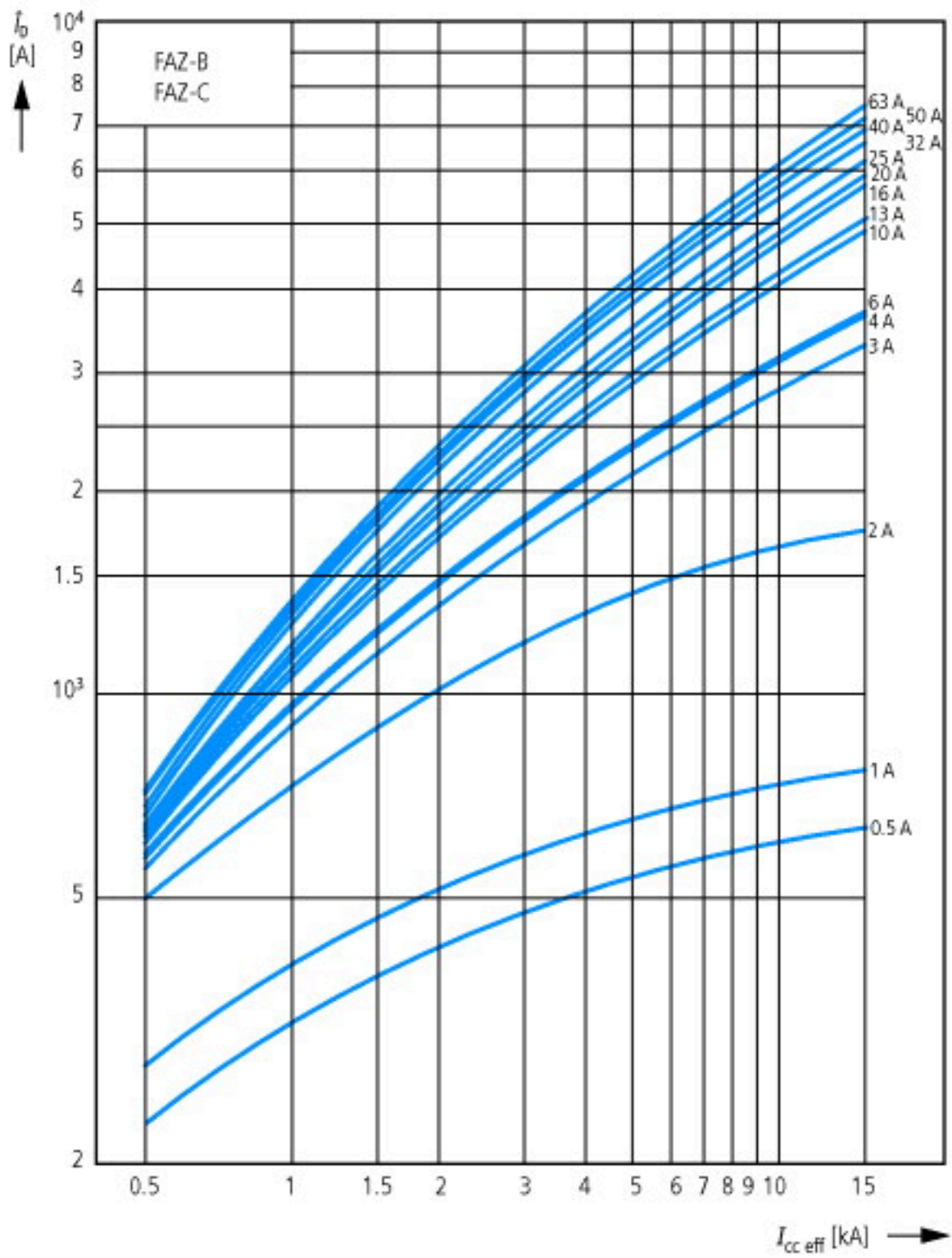
Durchlassstrom I_b Ermittlung nach IEC/EN 60898
