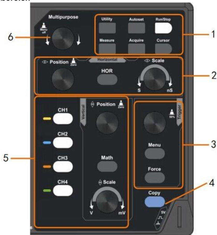
Abbildung 3 - 3 Übersicht über die Bedientasten
