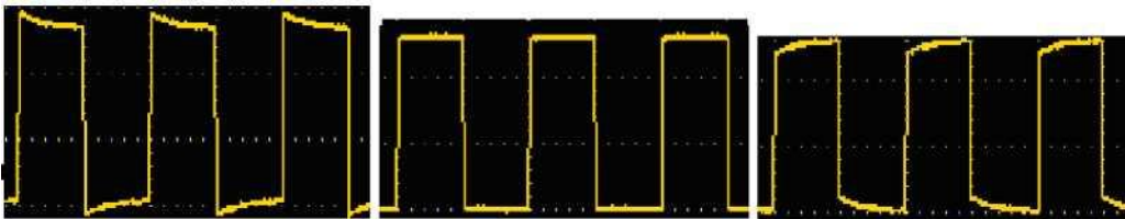
Abb. 3-6 Wellenformdarstellung der Tastkopfkompensation
