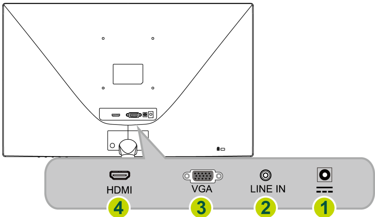
ABBILDUNG 2. ANSCHLISSEN AN EINEN PC
