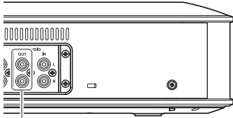
Audio-Ausgangsanschlüsse
