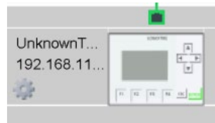
Gerät der Baureihe LOGO! TDE 6ED1055-4MH08-0BA0
