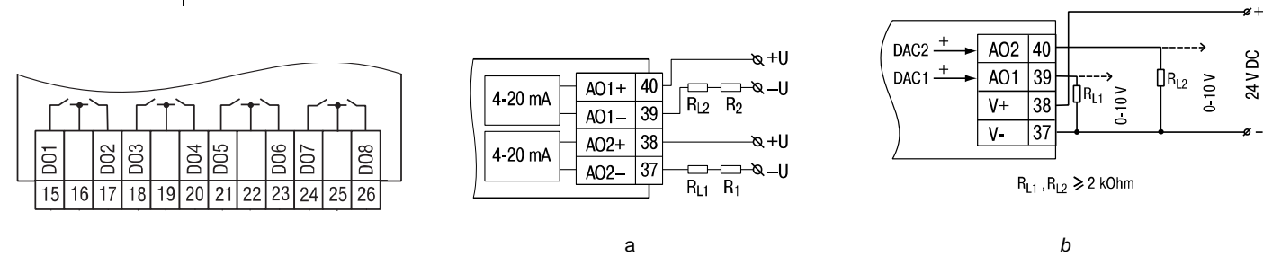
Abb. 8 Relaisausgänge
