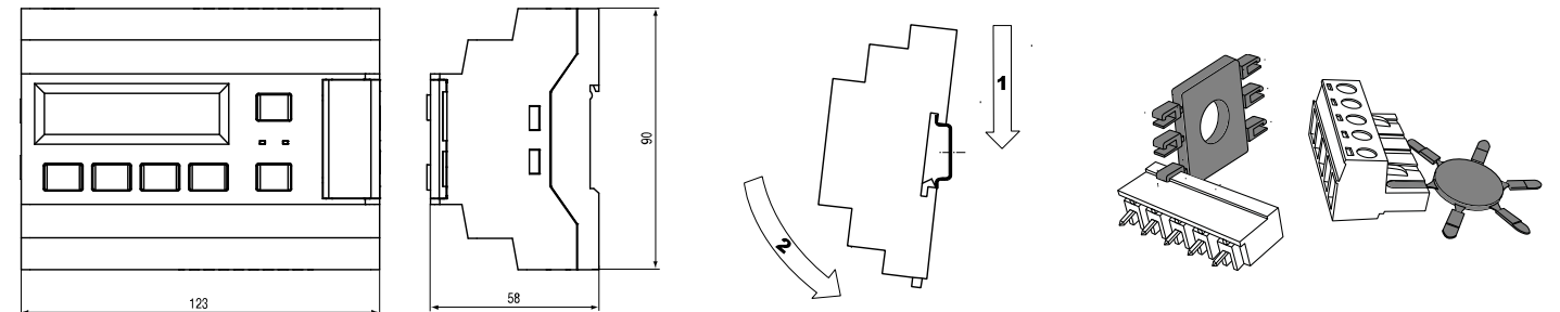
Abb. 1 Abmessungen
