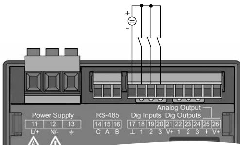
Abb. Anschluss digitalen Eingänge
