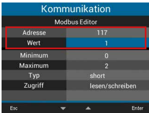
Abb. Fenster Kommunikation, Modbus-Editor (vgl. Tab. „Werte der Modbus-Adresse 117“)
