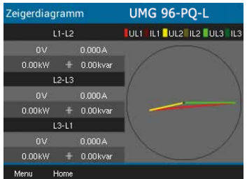
Zeigerdiagramm (Dreieck) (Dreiphasen-Dreileitersystem)
