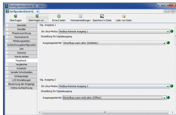
Abb. Konfiguration der digitalen Ausgänge als „Modbus Remote“ in Software GridVis®
