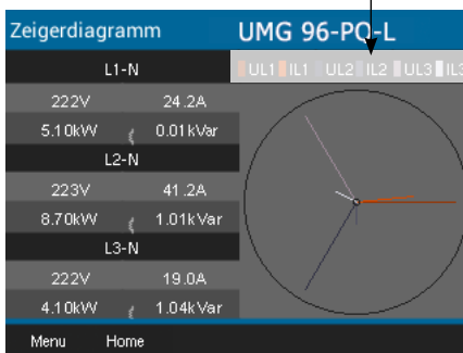
Abb. Fenster Zeigerdiagramm mit der Darstellung der Phasenreihenfolge entsprechend der Drehfeldrichtung.
