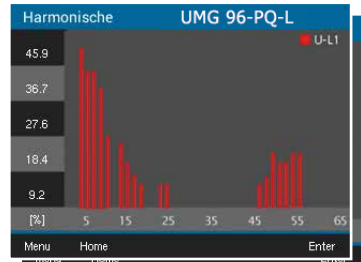
Anzeige der Harmonischen bis zur 65. (Spannung L1, L2, L3)
