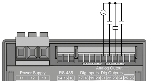
Abb. Anschluss Digital-/Impulsausgänge
