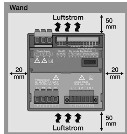
Abb. Einbaulage des UMG 96-PQ-L (Rückansicht)
