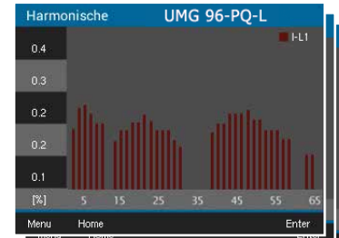
Anzeige der Harmonischen bis zur 65. (Strom L1, L2, L3)
