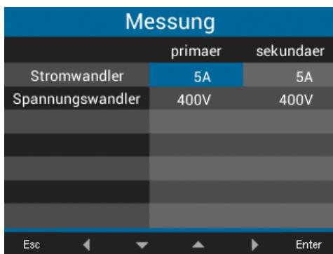
Abb. Fenster Messung mit den Einträgen zu den Messwandlern
