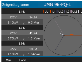
Zeigerdiagramm (Stern) (Dreiphasen-Vierleitersystem)
