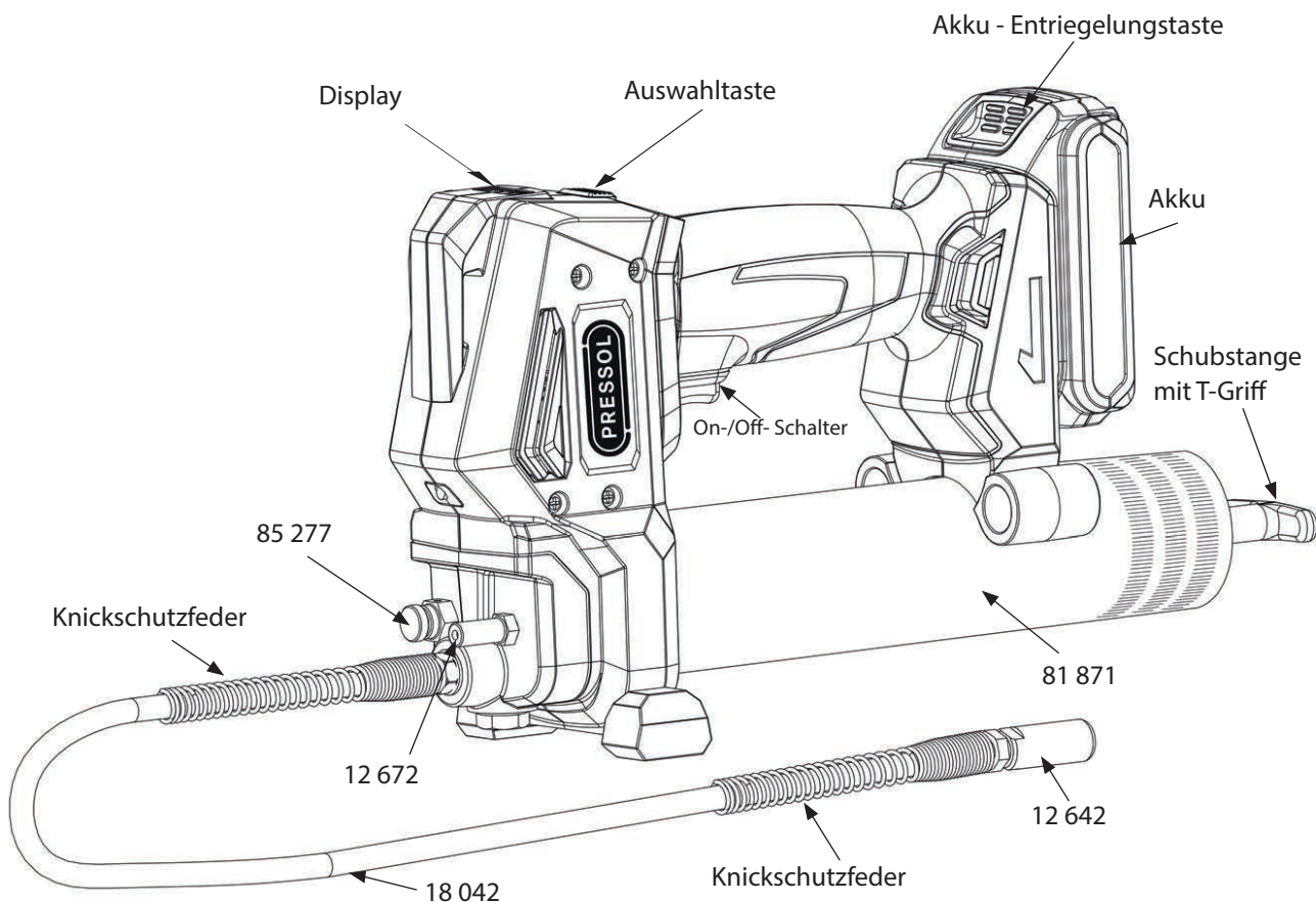
Abb. 3.2-1: Aufbau Akku-Fettpresse
