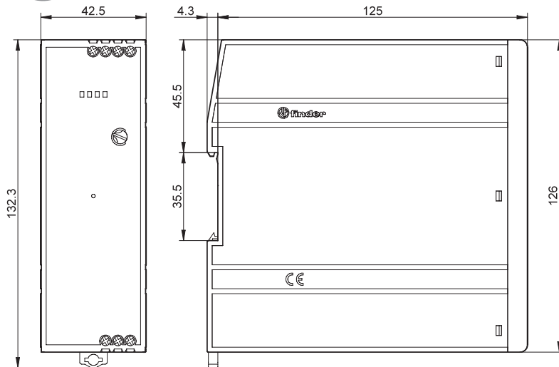
Typ 78.2A Käfigklemmen
