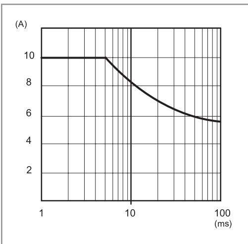
P78-7 Einschaltspitzenstrom-Belastbarkeit (78.1B)
