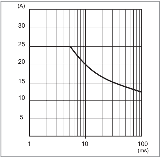
P78-9 Einschaltspitzenstrom-Belastbarkeit (78.2A)
