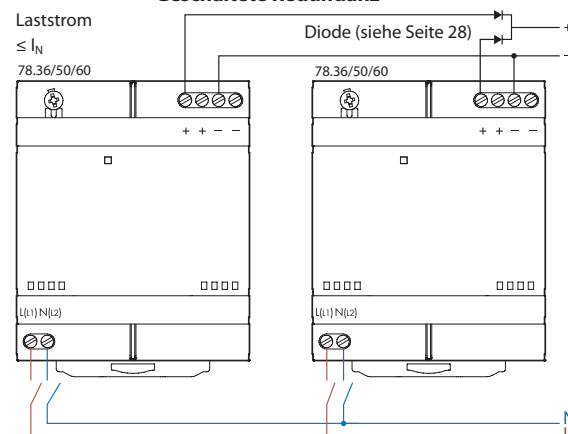
Geschaltete Redundanz
