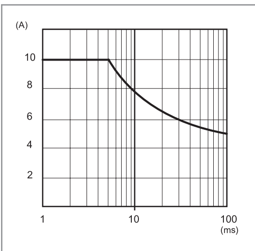
P78-8 Einschaltspitzenstrom-Belastbarkeit (78.1D)
