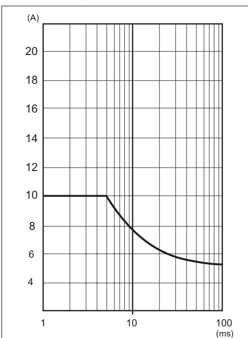
P78-8 Einschaltspitzenstrom-Belastbarkeit (78.1D)
