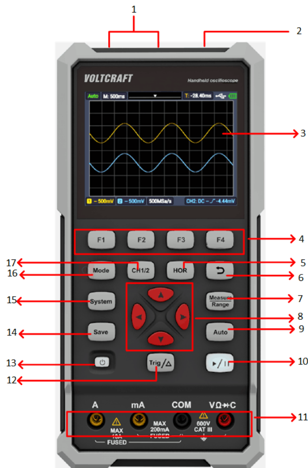
Abbildung 3-1: Vorderseite des Oszilloskops
