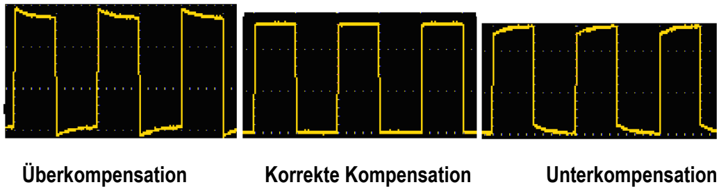
Abbildung 3-4: Anzeige der Wellenform der Prüfspitzenkompensation
