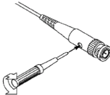
Abbildung 3-5: Prüfspitzenabgleich
