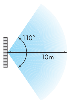
Waagrechter Erfassungsbereich
