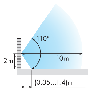
Senkrechter Erfassungsbereich
