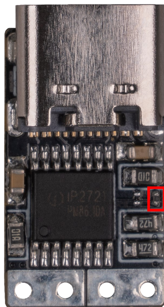
Rechter Widerstand eingelötet = 20 V
