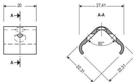
APESCLIP
