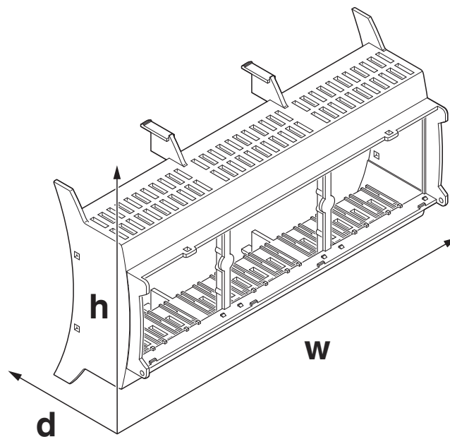
Maßzeichnung
