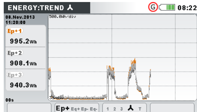
Abbildung 4.29: Bildschirm Energietrend
