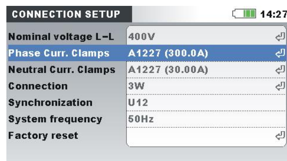
Abbildung 5.19: Automatisch erkannte Einstellungen für die Stromzangen
