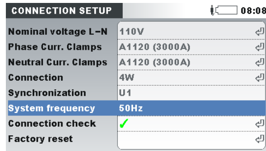
Abbildung 5.2: Menü Anschlusseinrichtung
