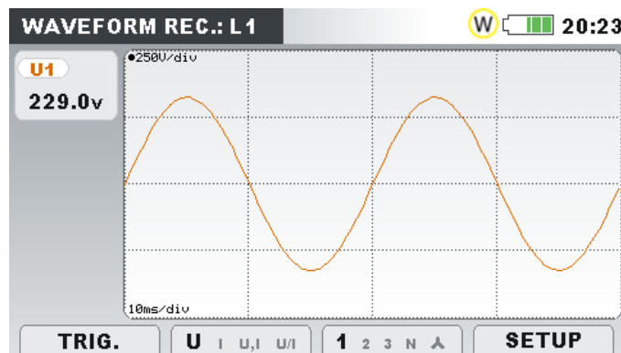
Abbildung 4.51: Wellenformrekordererfassungs-Bildschirm
