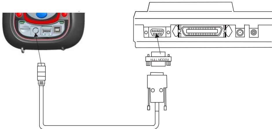
Abbildung 5.21: Anschließen des Druckers DPU 414 am Gerät
