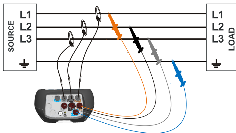
Abbildung 5.6: Dreiphasiges 3-Leitersystem
