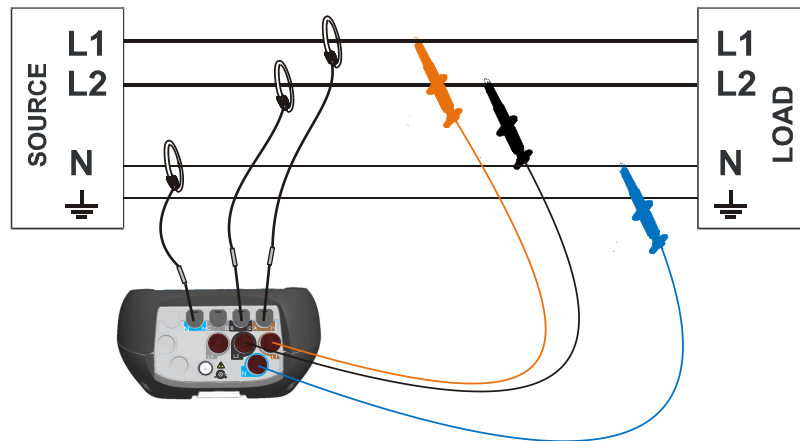
Abbildung 5.12: Zweiphasiges 4-Leitersystem
