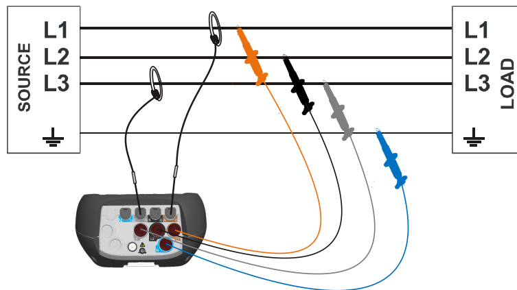
Abbildung 5.8: Offenes Dreieck-3-Leitersystem (Aaronschaltung)
