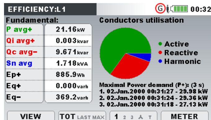
Abbildung 4.30: Bildschirm Energieeffizienz
