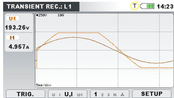
Abbildung 4.54: Transientenrekordererfassungsbildschirm
