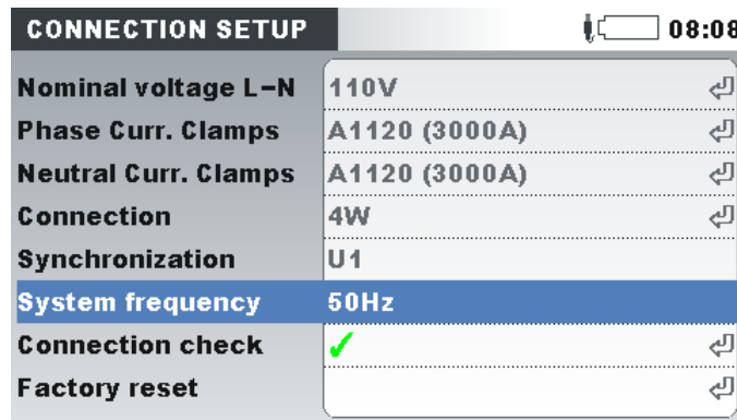
Abbildung 4.67: Bildschirm „ANSCHLUSSEINRICHTUNG“
