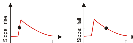
Abbildung 6.26: Triggergradient
