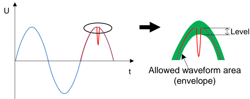
Abbildung 6.27: Transientenauslöserdetektion (Hüllkurve)
