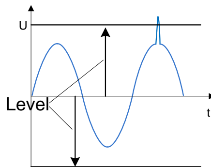
Abbildung 6.28: Transientenauslöserdetektion (Hüllkurve)
