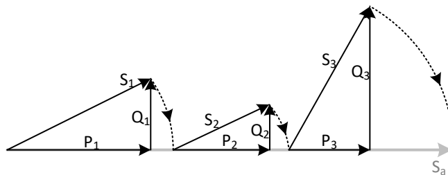
Abbildung 146: Arithmetische Darstellung der Gesamtleistungsrechnung
