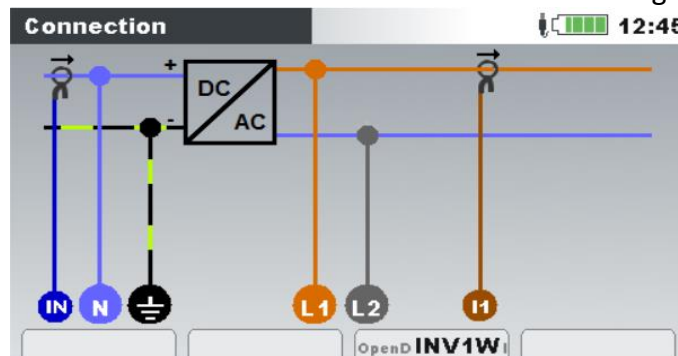
Abbildung 108: Auswählen des einphasigen Wechselrichtersystems auf dem Gerät
