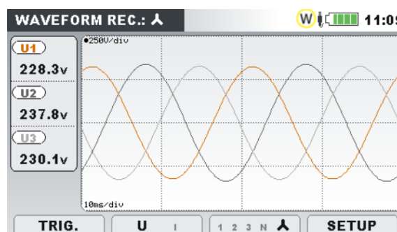
Abbildung 59: Oszilloskop-Bildschirm des Wellenform-Rekorders
