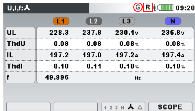
Abbildung 76: Bildschirm von der U,I,f-Messung in der aufgerufenen Momentaufnahme
