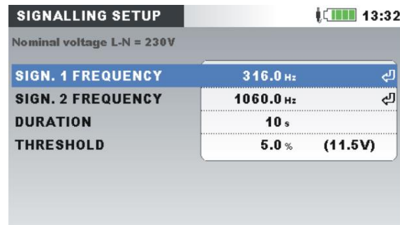
Abbildung 81: Bildschirm zur Netzsignaleinrichtung
