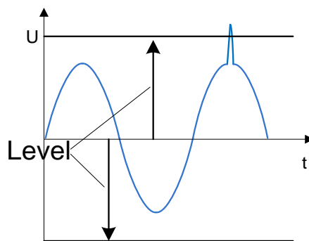
Abbildung 169: Feststellung des Transienten-Auslösers (Niveauschwelle)
