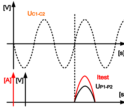
Abbildung 6.5: Beispiele für die Spannungs- und Strom-Wellenform bei Hochstrom-Messung
