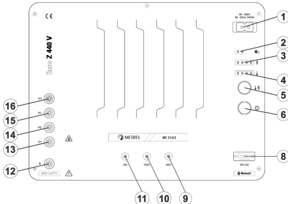
Abbildung 3.1: Bedienfeld
