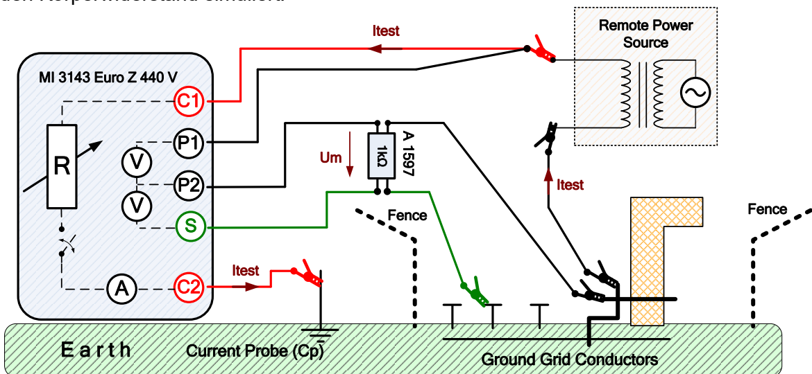
Abbildung 6.7: Beispiel für eine U_Touch-Messung
