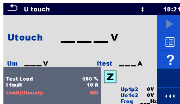
Abbildung 6.90: Berührungsspannungsmenü
