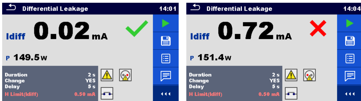
Abbildung 6.44: Beispiele für Ergebnisse der Differenzstrom Messung
