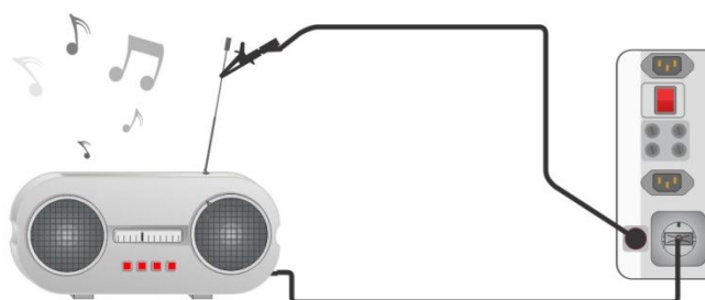
Abbildung 6.49: Berührungsableitstrom Prüfverbindungen
