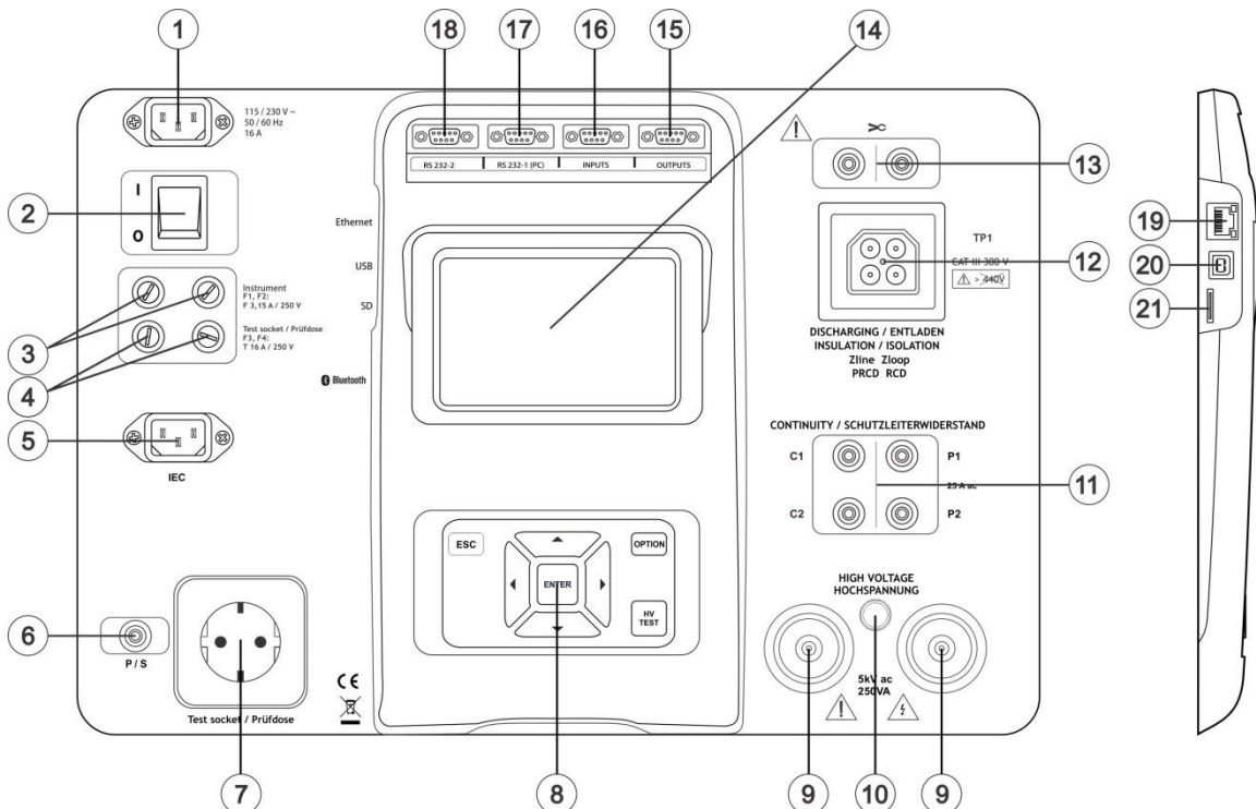
Abbildung 3.1: Vorderseite
