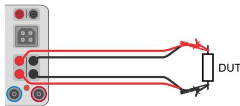
Abbildung 6.19: Widerstandsmessung 4 - Leiter
