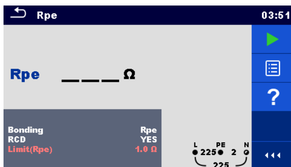
Abbildung 6.108: Menü Schutzleiterwiderstandsmessung
