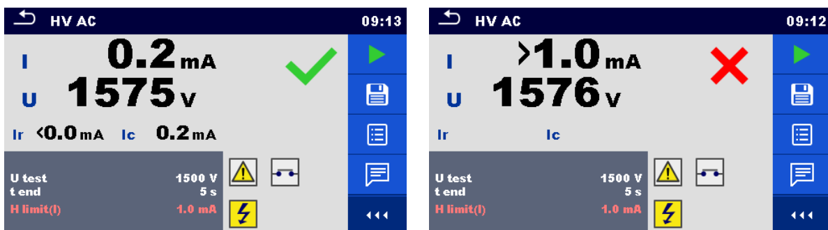
Abbildung 6.132: Beispiele für Ergebnisse der HV AC Prüfung
