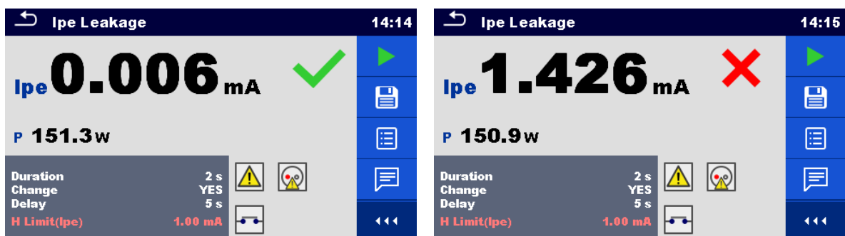
Abbildung 6.47: Beispiele für Ergebnisse Schutzleiterableitstrom Messung
