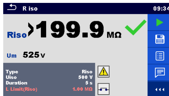
Abbildung 6.5: Einzelprüfung Ergebnisbildschirm
