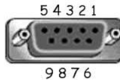
Abbildung 8.7: Ausgangsbuchse - Pinbelegung
