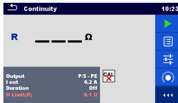
Abbildung 6.16: Menü RPE-Widerstandsmessung
