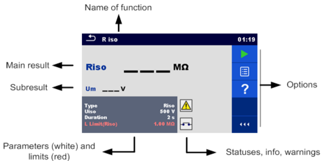
Abbildung 6.1: Aufbau Einzelprüfungsbildschirm
