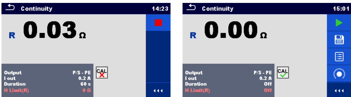
Abbildung 6.23: Unkompenziertes und kompenziertes Ergebnis
