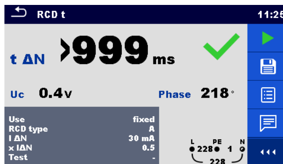
Abbildung B.5: Beispiel für das Ergebnis der Auslözeitmessung mit Phase zufällig aktiviert
