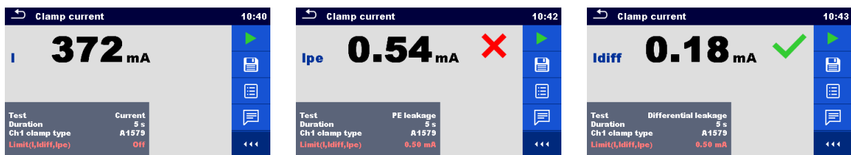
Abbildung 6.143: Beispiele für Ergebnisse der Stromzangenmessung
