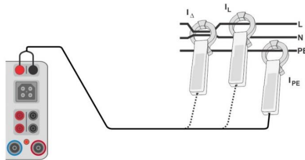
Abbildung 6.142: Zangenstrom Prüfverbindungen
