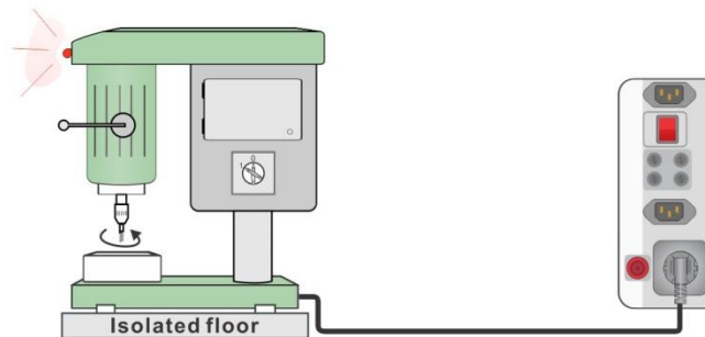
Abbildung 6.46: Schutzleiterableitstrom
