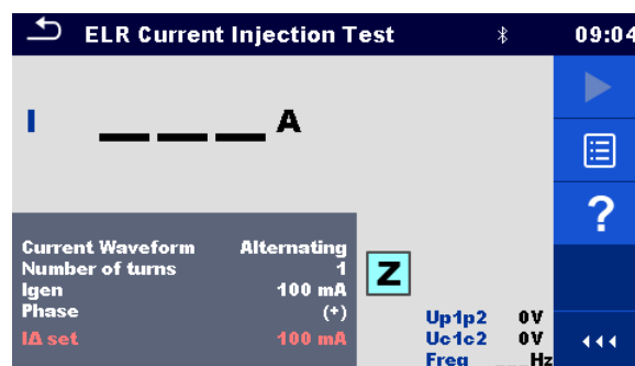
Abbildung 6.95: ELR-Stromeinspeisungstest Menü
