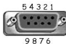
Abbildung 8.6: Eingangsbuchse - Pinbelegung
