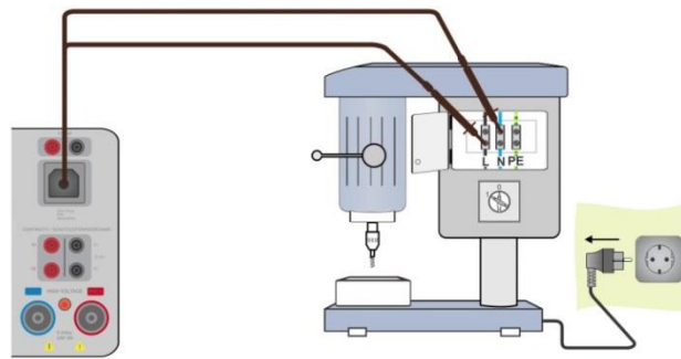
Abbildung 6.148: Messung Entladezeit
