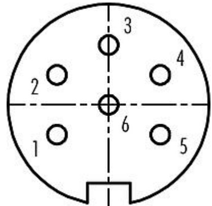
Polbild (Steckseite)
