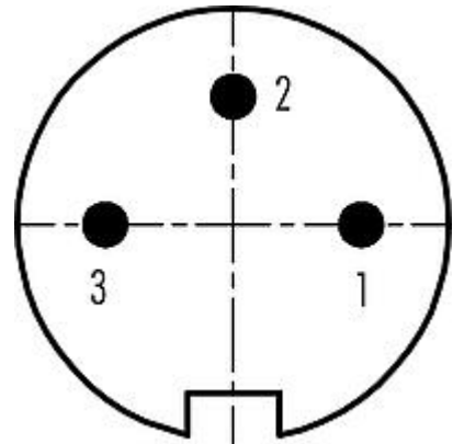
Polbild (Steckseite)
