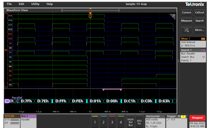
Triggerung und Dekodieren von digitalen Kanälen
