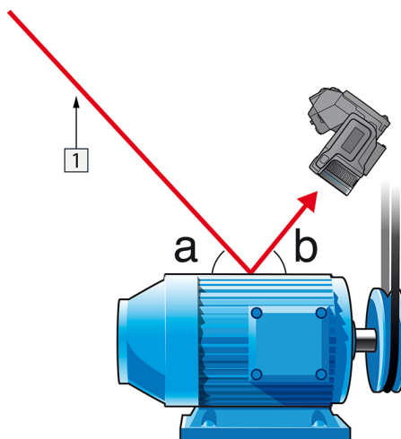
Abbildung 33.1 1 = Reflektionsquelle
