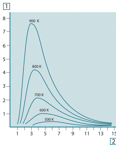
Abbildung 36.4 Die spektrale Abstrahlung eines schwarzen Körpers gemäß dem Planckschen Gesetz, für verschiedene absolute Temperaturen dargestellt. 1: Spektrale Abstrahlung ( \text{W}/\text{cm}^2 \times 10^3(\mu\text{m}) ); 2: Wellenlänge ( \mu\text{m} )
