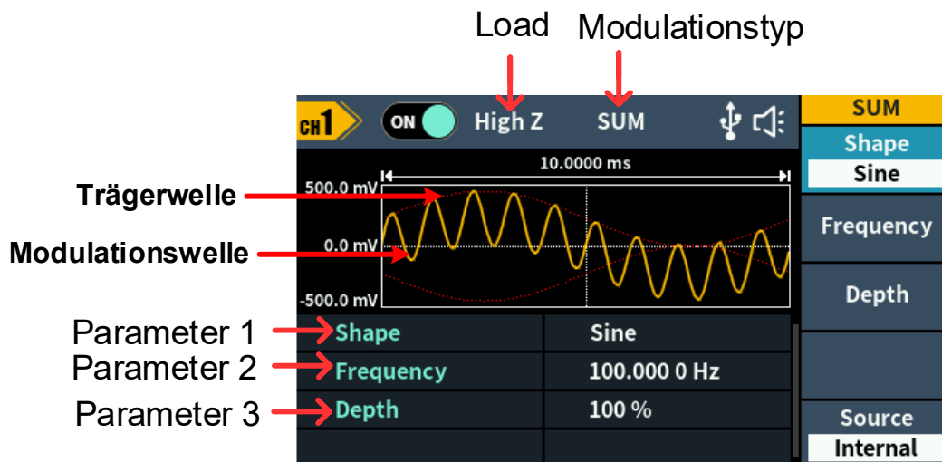
Abbildung 5-27: SUM-Benutzeroberfläche
