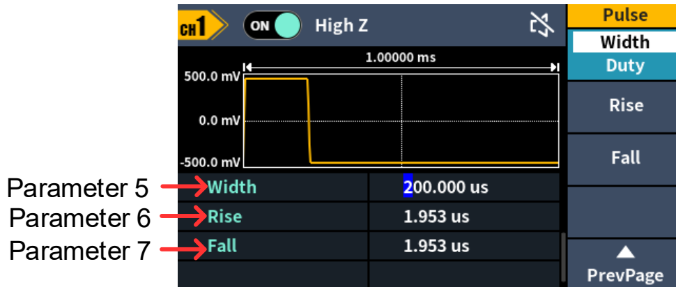
Abbildung 5-7: Benutzeroberfläche der Impulswelle
