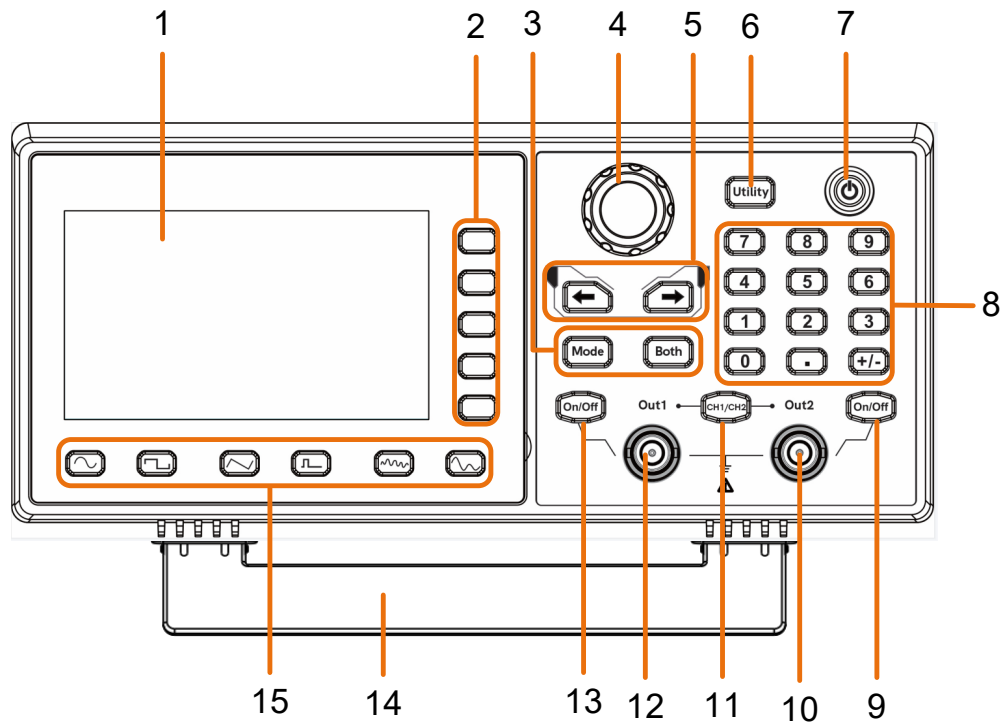
Abbildung 4-1: Gerätefront
