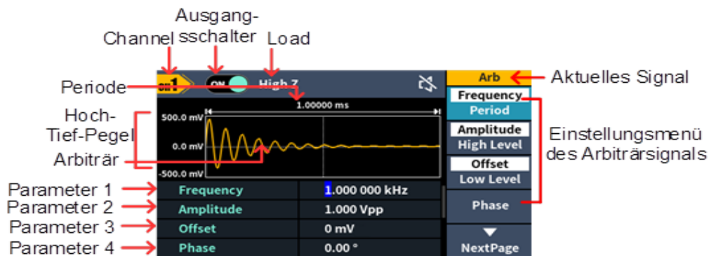
Abbildung 5-10: Benutzeroberfläche der Arbiträr-Wellenform
