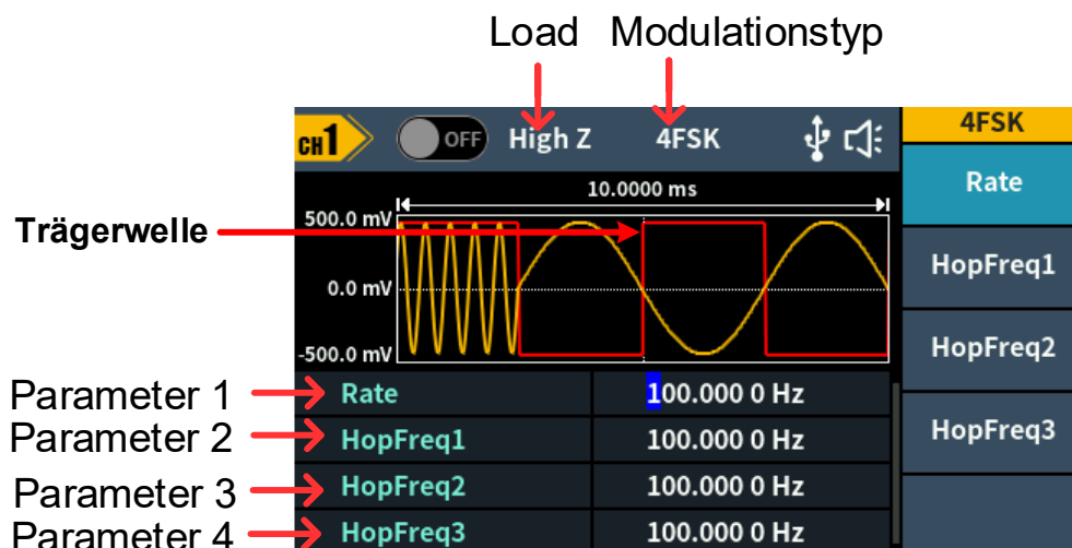
Abbildung 5-23: 4FSK-Benutzeroberfläche
