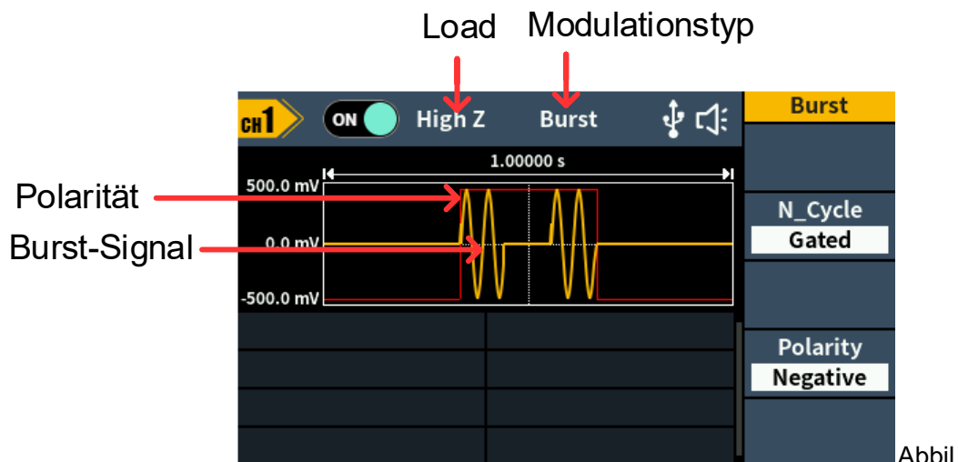
Abbildung 5-12: Benutzeroberfläche N-Zyklus-Burst
