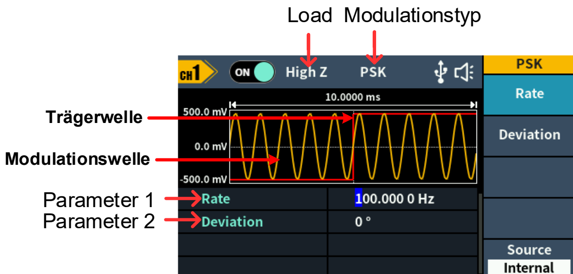
Abbildung 5-20: PSK-Benutzeroberfläche
