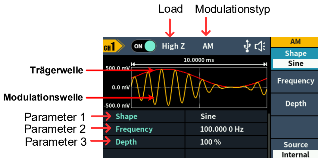
Abbildung 5-14: AM-Benutzeroberfläche
