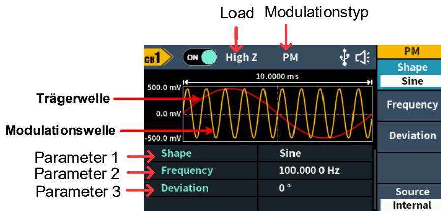
Abbildung 5-17: PM-Benutzeroberfläche
