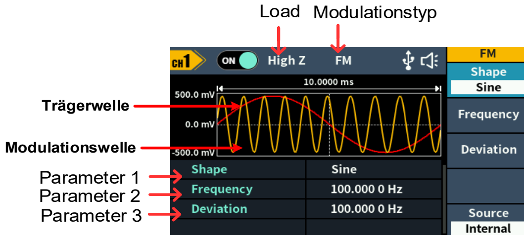
Abbildung 5-16: FM-Benutzeroberfläche
