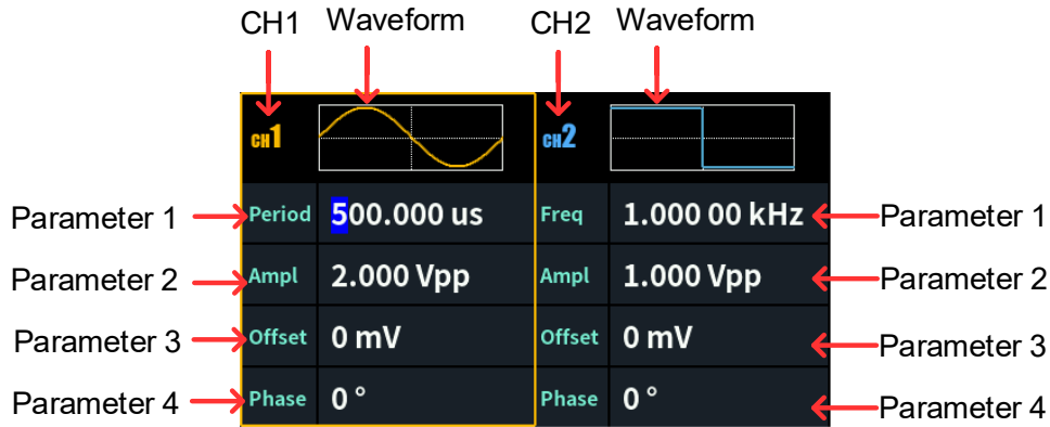
Abbildung 5-1: Benutzeroberfläche der Taste (Both)
