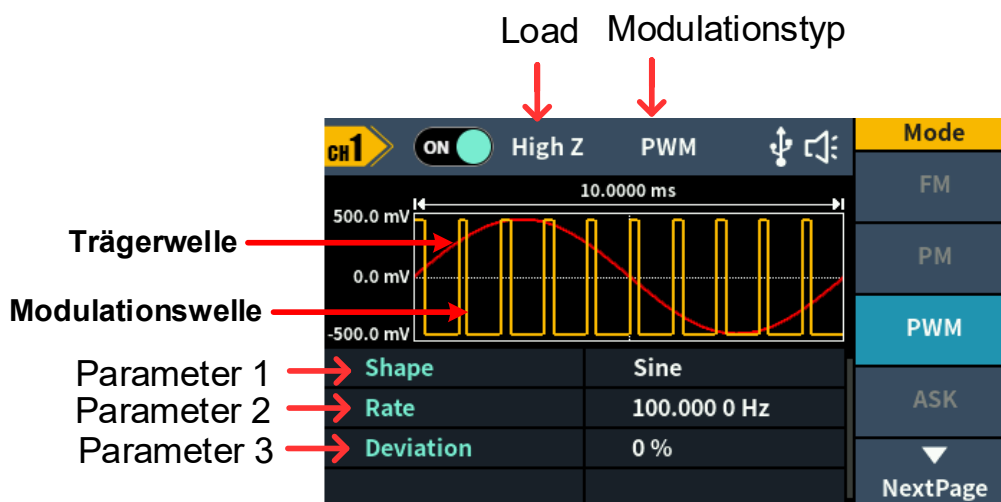
Abbildung 5-18: PWM-Benutzeroberfläche
