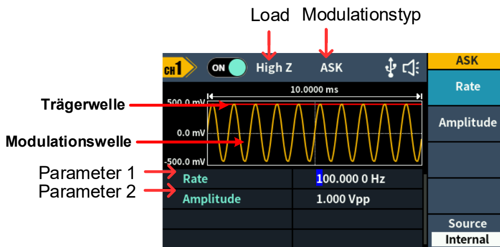
Abbildung 5-19: ASK-Benutzeroberfläche
