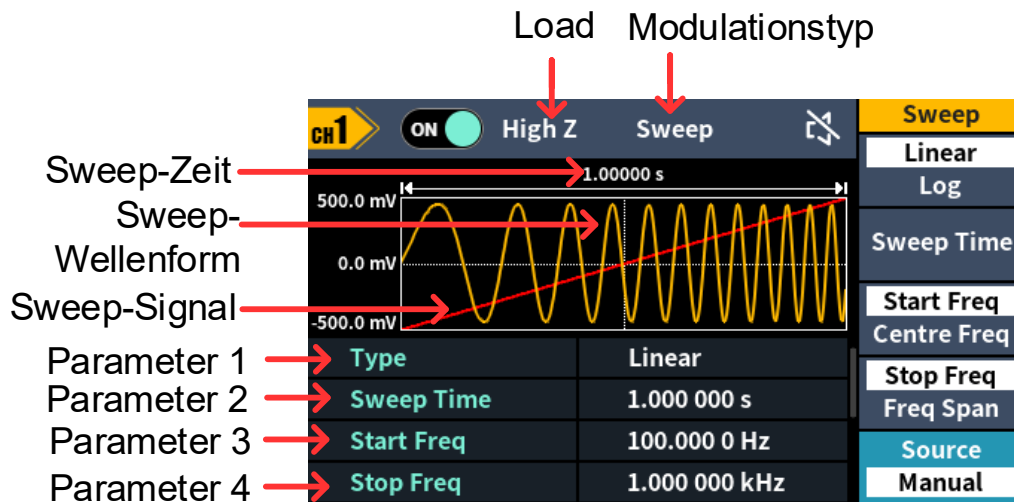
Abbildung 5-11: Benutzeroberfläche des Sweep-Modus
