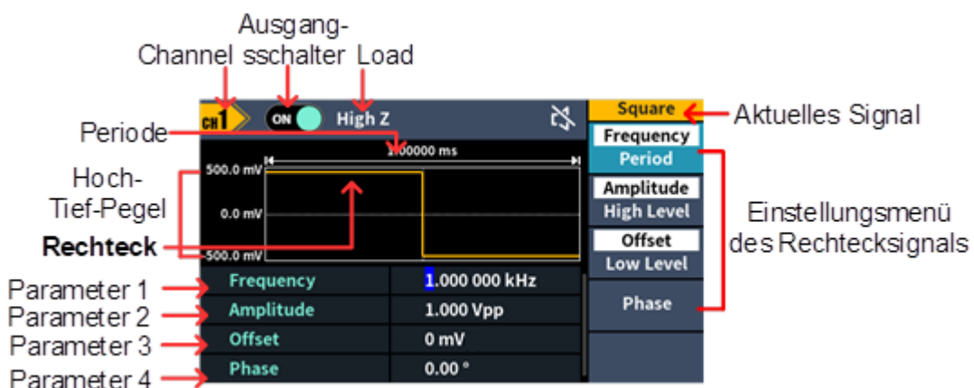
Abbildung 5-4: Benutzeroberfläche der Rechteckwelle
