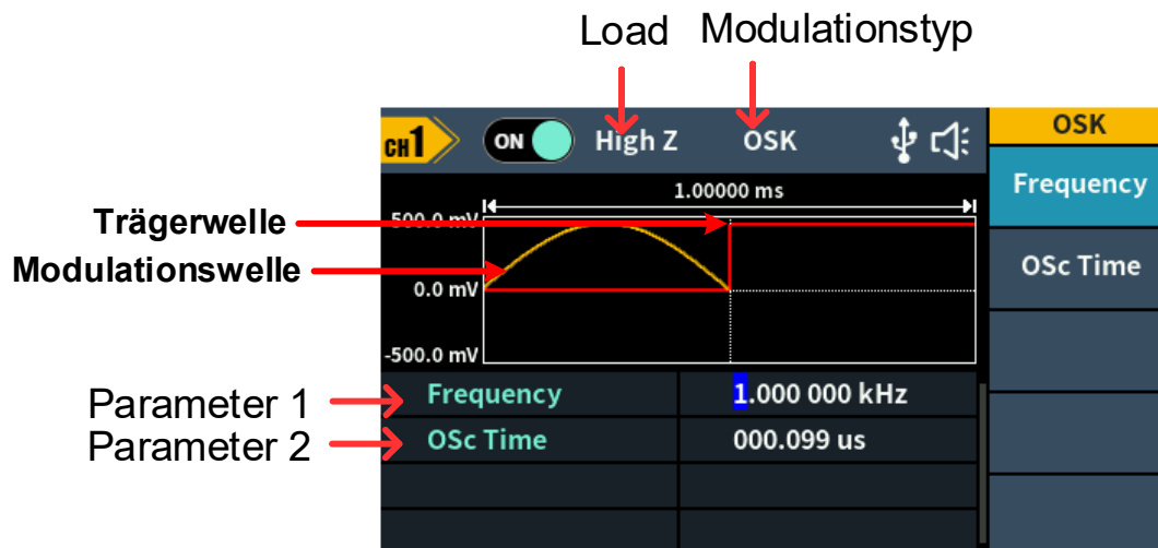
Abbildung 5-26: OSK-Benutzeroberfläche
