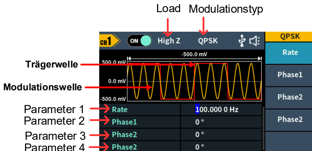
Abbildung 5-25: QPSK-Benutzeroberfläche
