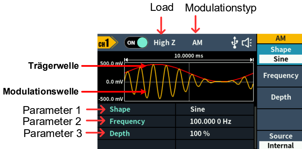
Abbildung 5-13: Benutzeroberfläche Gated Burst
