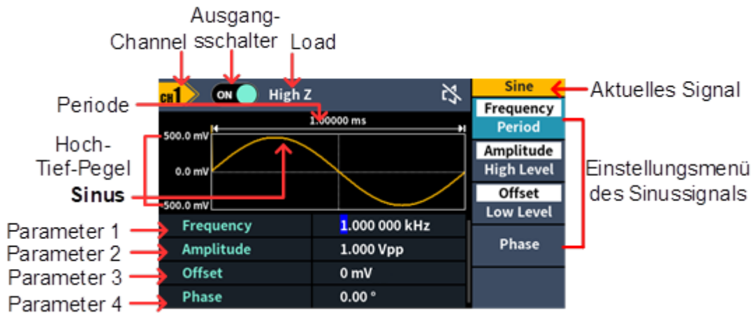
Abbildung 5-2: Benutzeroberfläche der Sinuswelle
