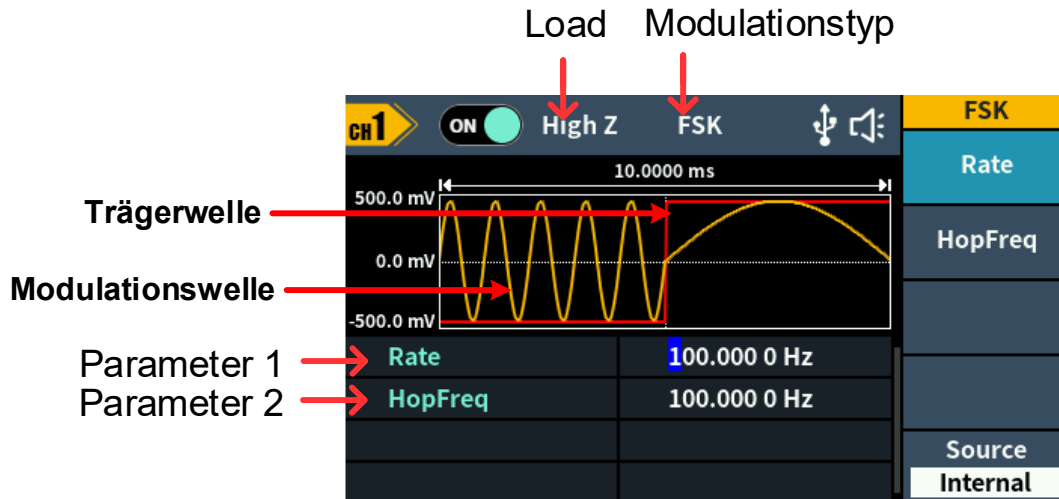
Abbildung 5-21: FSK-Benutzeroberfläche
