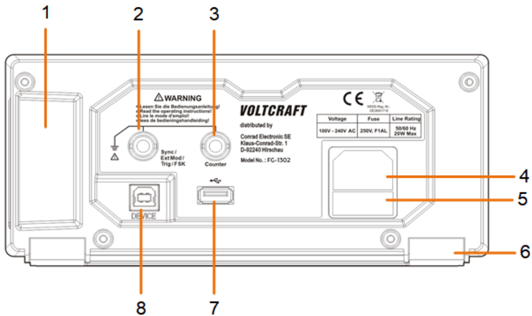
Abbildung 4-2: Geräterückseite
