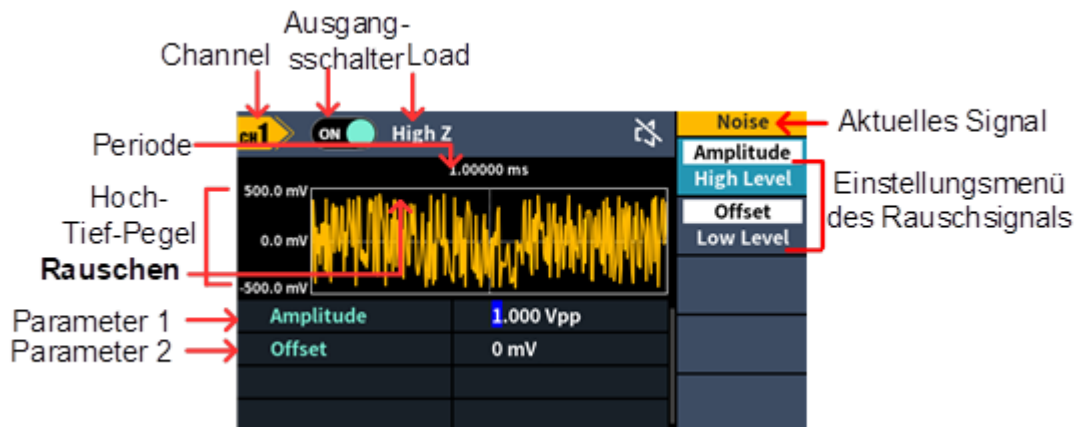
Abbildung 5-9: Benutzeroberfläche der Rauschwelle
