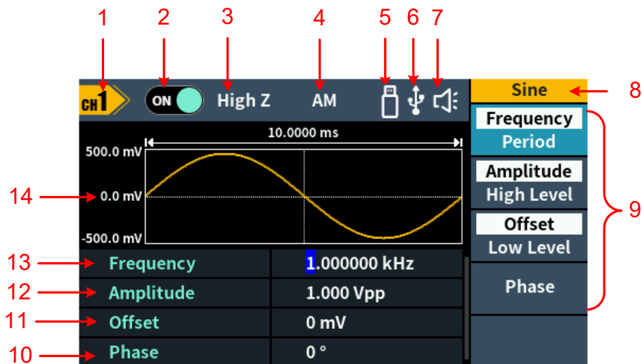
Abbildung 4-3: Benutzeroberfläche
