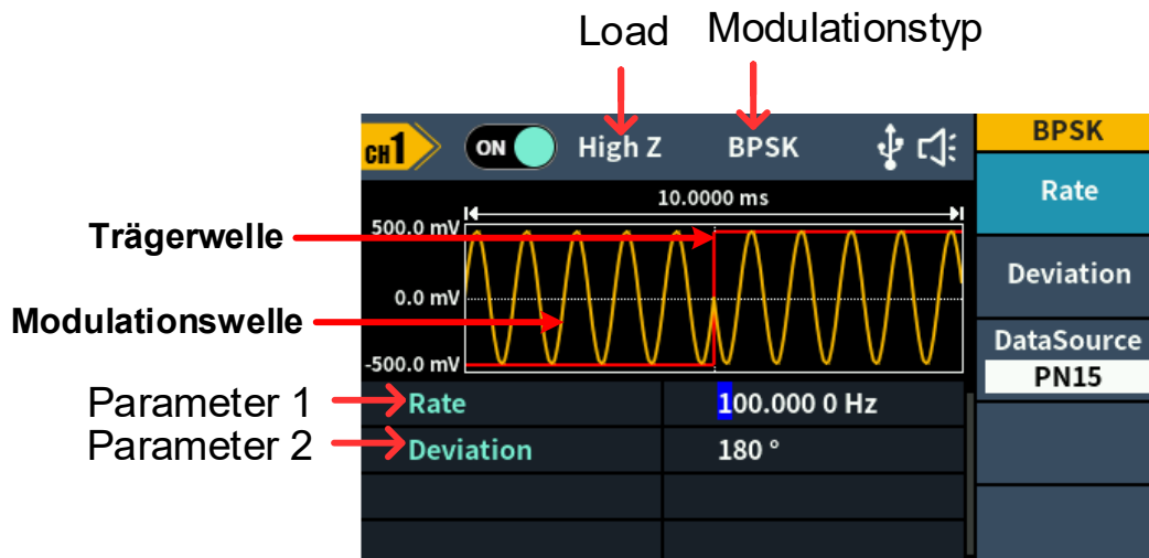
Abbildung 5-24: BPSK-Benutzeroberfläche
