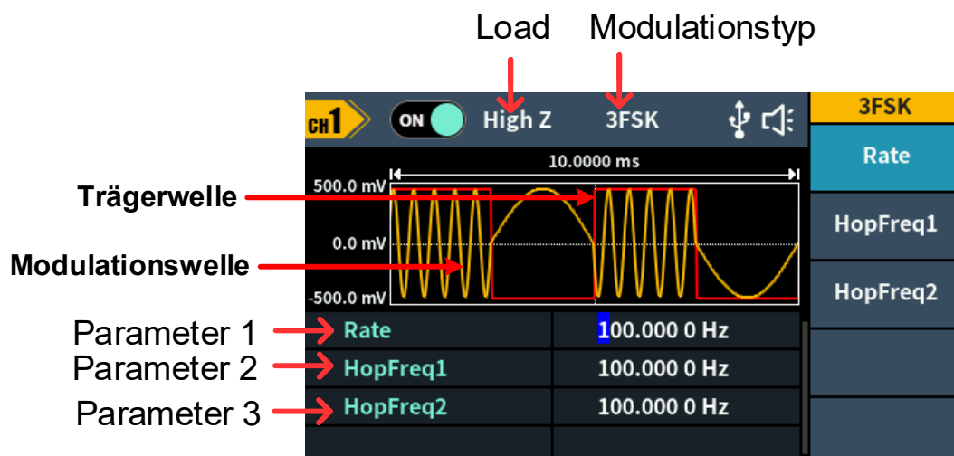
Abbildung 5-22: 3FSK-Benutzeroberfläche
