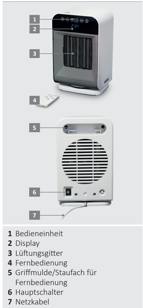
Abb.1: Geräteübersicht
