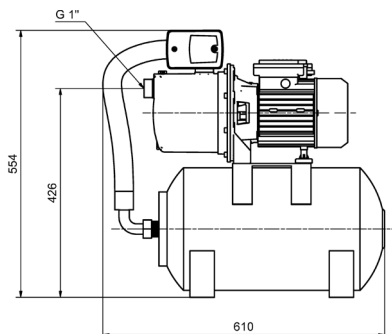
GARDEN 2000 mit ZPC 01 und Membranausdehnungsgefäß aus Stahl
