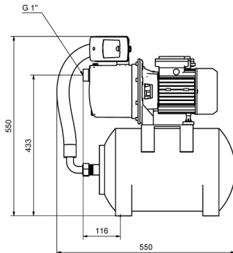
GARDEN 2000 mit ZPC 01 und Membranausdehnungsgefäß aus Edelstahl
