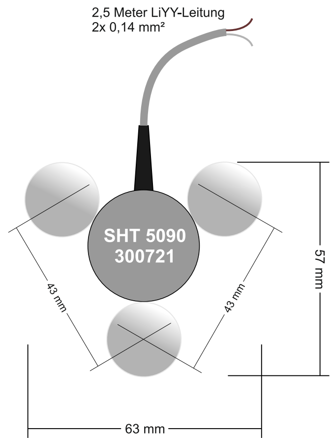
43 mm Kugelabstand entspricht ~21,5 mm einfachem Kontaktabstand ► mind. 30 µS Leitfähigkeit für SHT 5000, 5001, 5002
