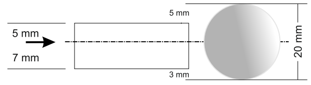
asymmetrische Bohrung = 3 oder 5 mm Bodenfreiheit Kugeln aus V2A Edelstahl blank gedreht, Werkstoff 1.4301
