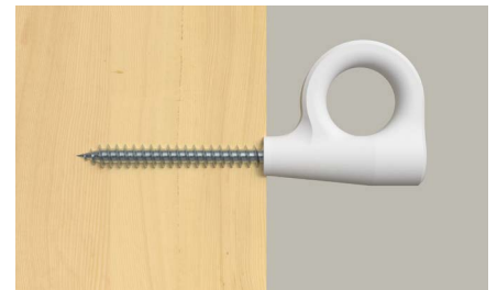
Um einen geringeren Wandabstand zu erreichen, kann der Haken ohne Schaftbereich montiert werden. Brechen Sie dazu den vorderen Teil einfach von Hand ab.
