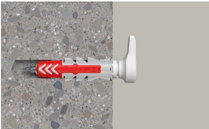
In Vollstein erreicht der EasyHook seine höchsten Lastwerte.
