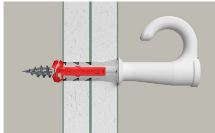
In Kombination mit dem DuoPower kann der EasyHook in einfach und doppelt beplankten Gipskartonplatten eingesetzt werden.
